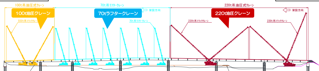
パネル敷設側面図
