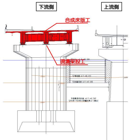
断面図
