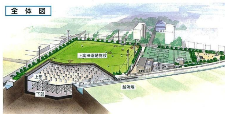
図2-5 上高田調節池 全体図
