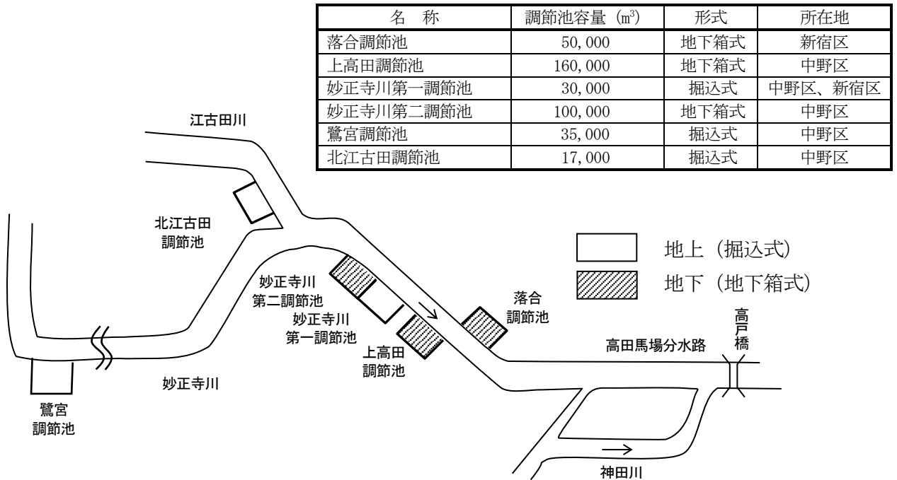
図2-4 妙正寺川・江古田川の調節池
