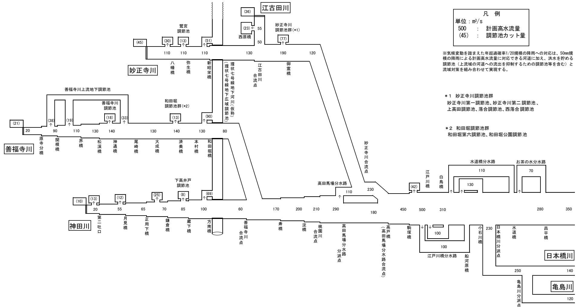
図 3-1 計画流量配分図
