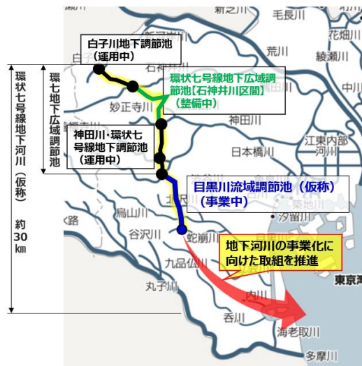
図4-10 環状七号線地下河川（仮称）全体図
