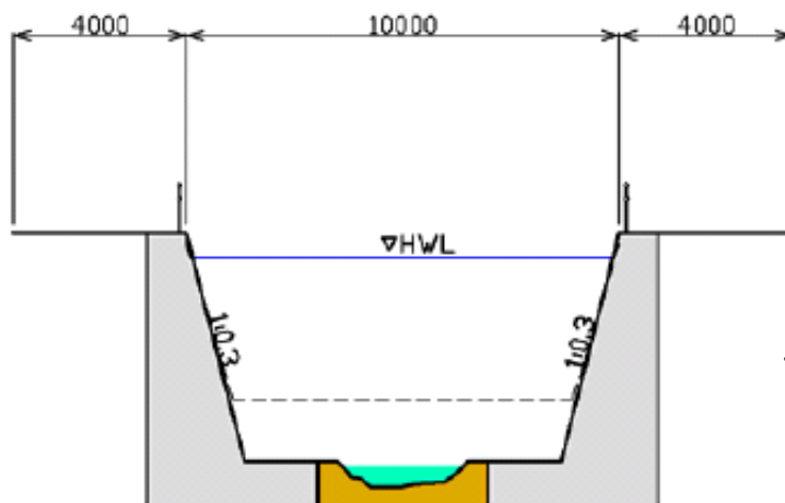
図 4-1 標準断面図 (神田川)
