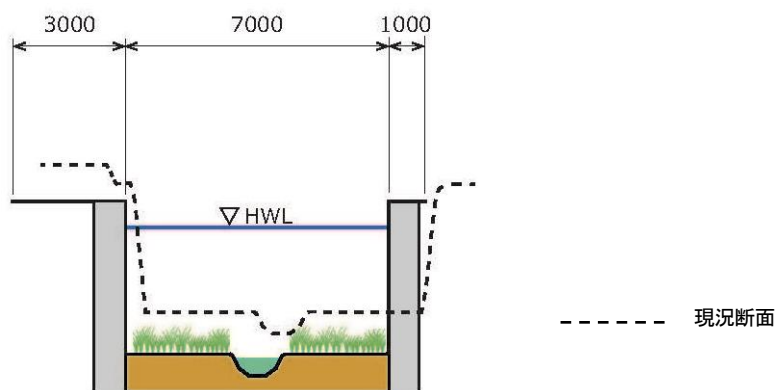
图 4-4 標準断面图 (江古田川)
