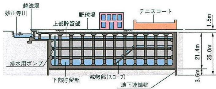
図2-6 上高田調節池 断面図
