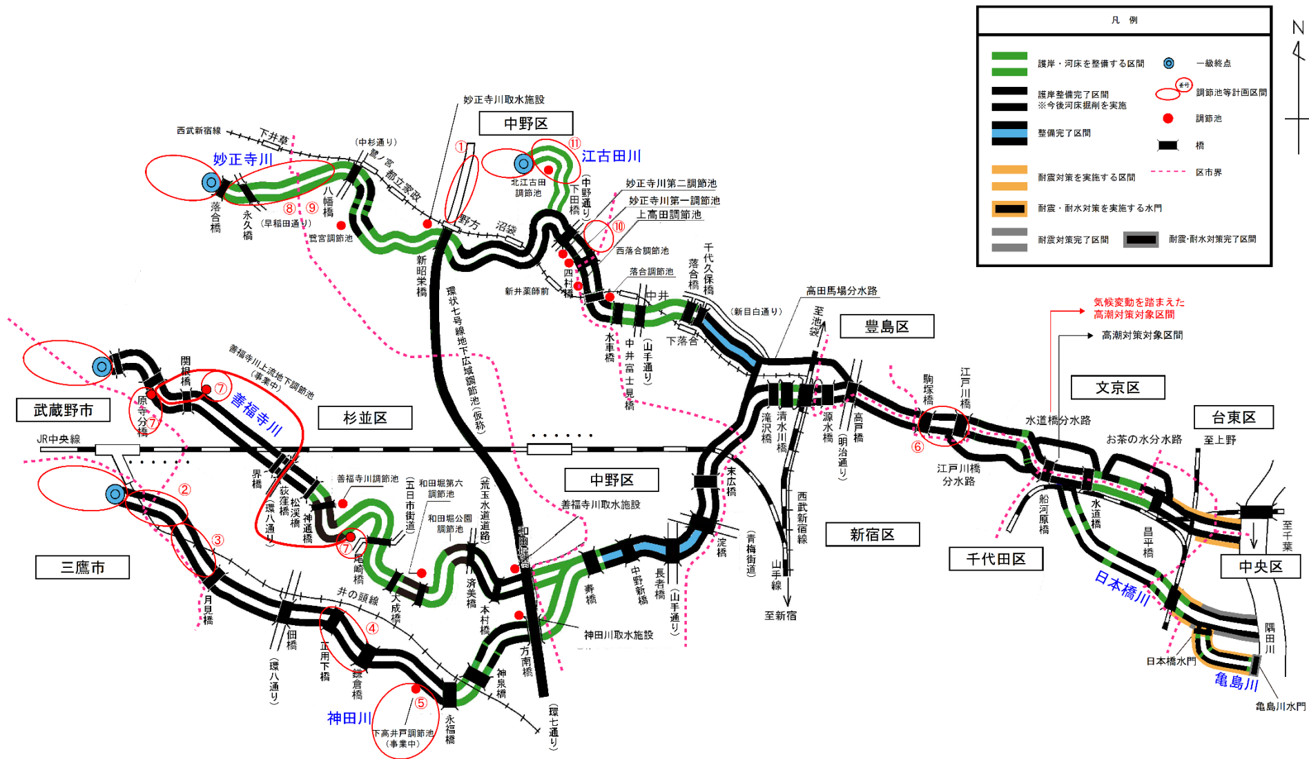
図4-5 神田川流域 河川整備箇所図
