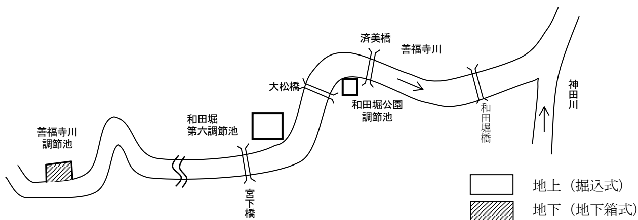
図 2-7 善福寺川の調節池
