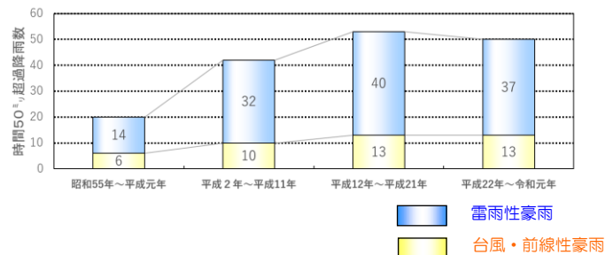
図 1-5 1時間50mm又は24時間152mmを超過する 発生要因別降雨数の経年変化 (昭和55年~令和元年(過去40年間))
