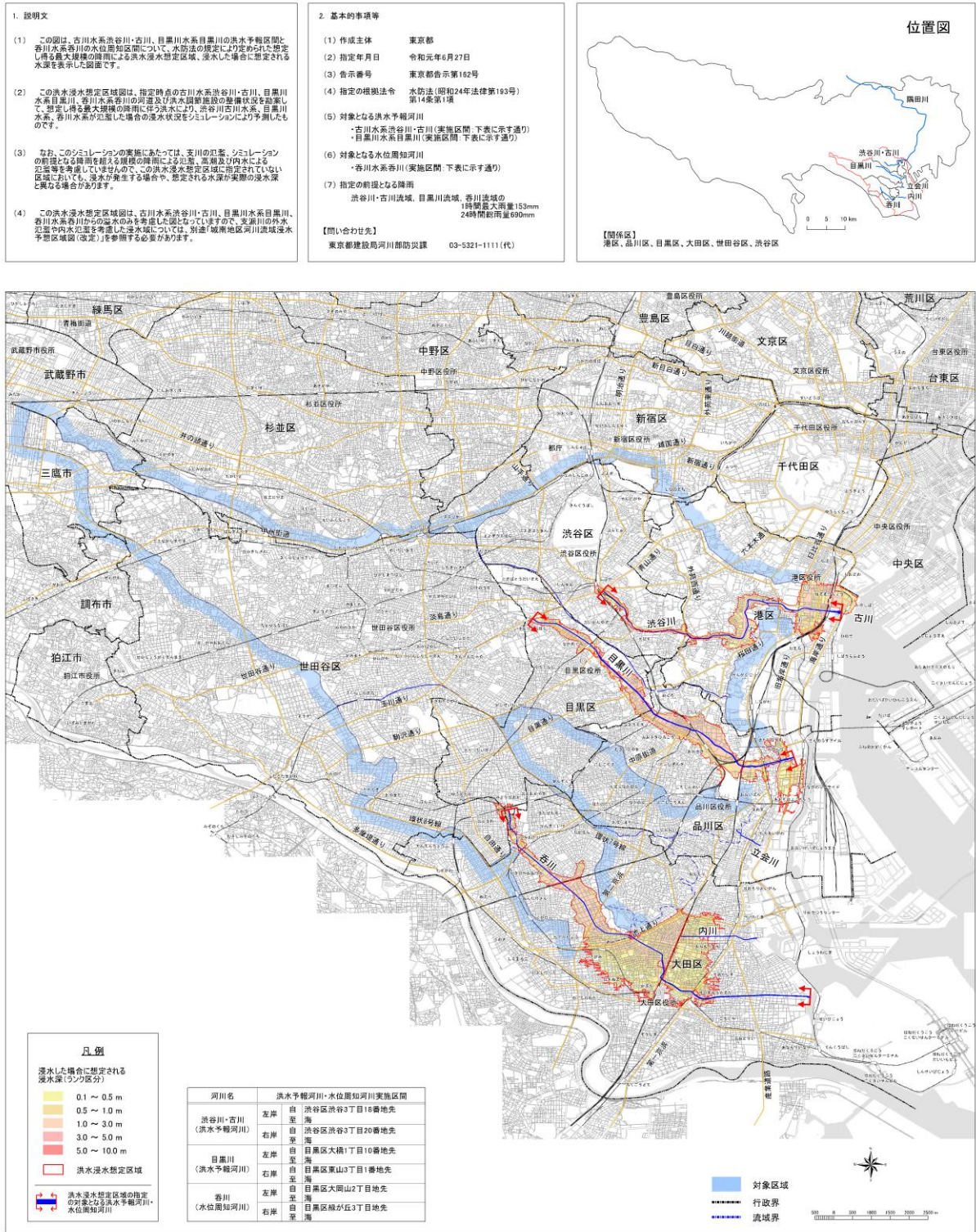
図5-2 古川水系渋谷川・古川、目黒川水系目黒川、呑川水系呑川 洪水浸水想定区域図(想定最大規模)(令和元年6月公表)
