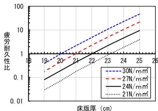
図-13 床版厚と圧縮強度と疲労耐久性の関係
