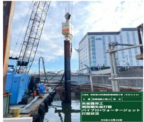
②吐口側鋼矢板打設
