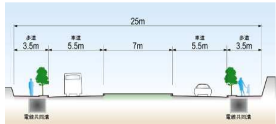
標準断面図
