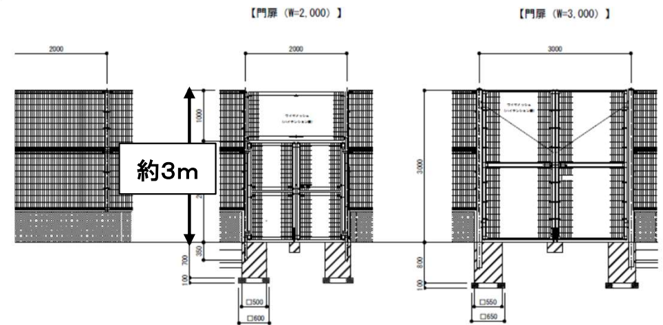
フェンス詳細図
