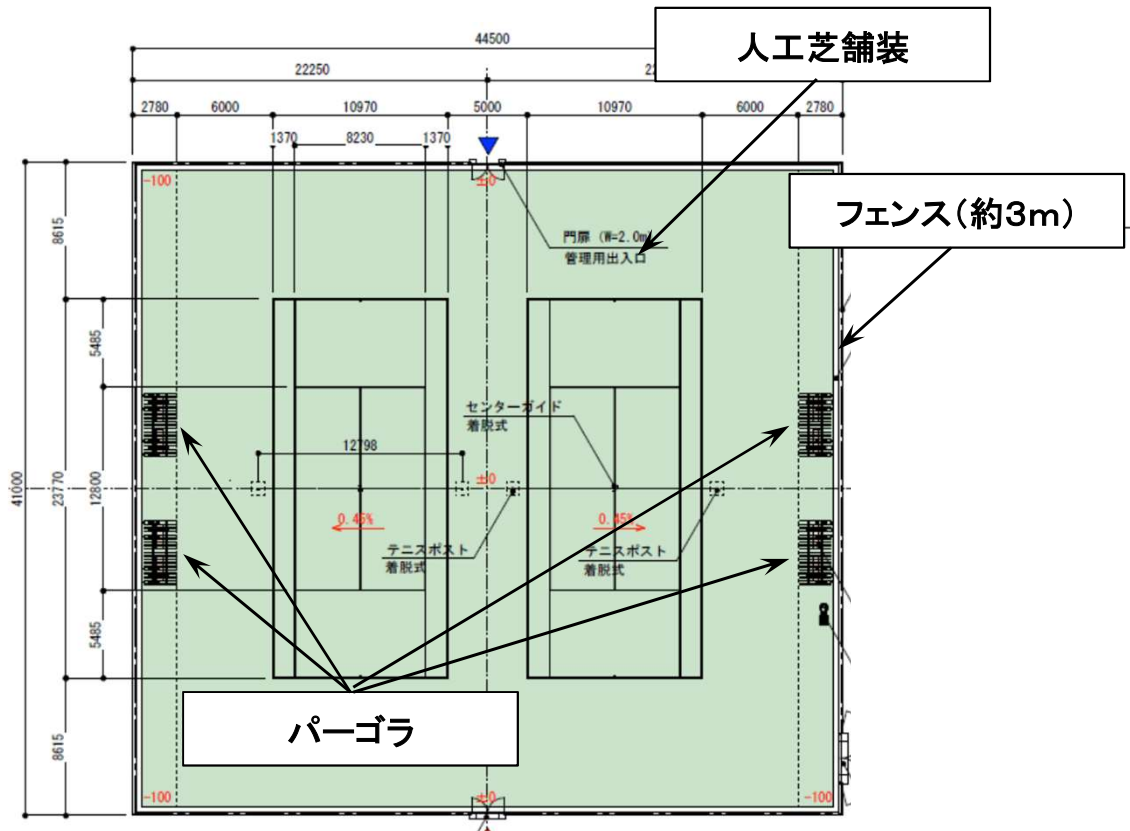
テニスコート平面図
