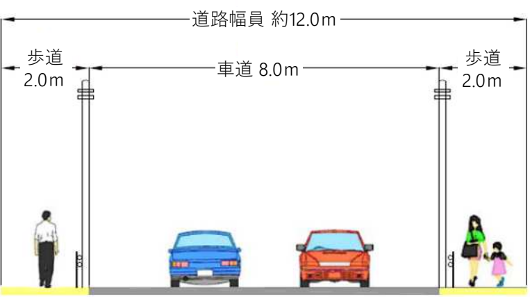
標準断面図 (現況)
