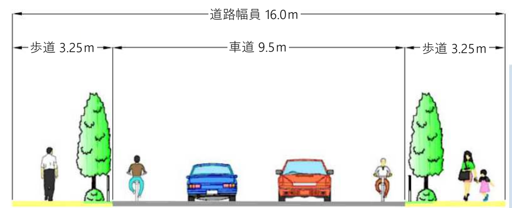
標準断面図 (計画)
