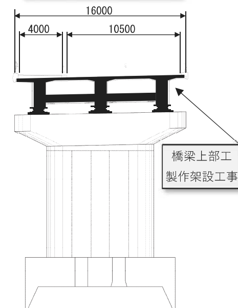
断面図(新設下流橋)
