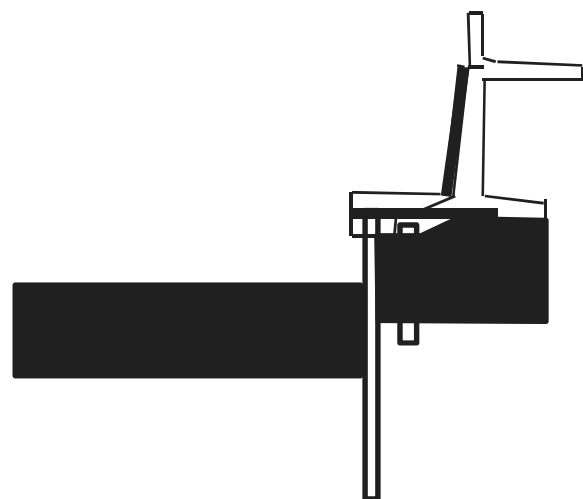
標準断面図
