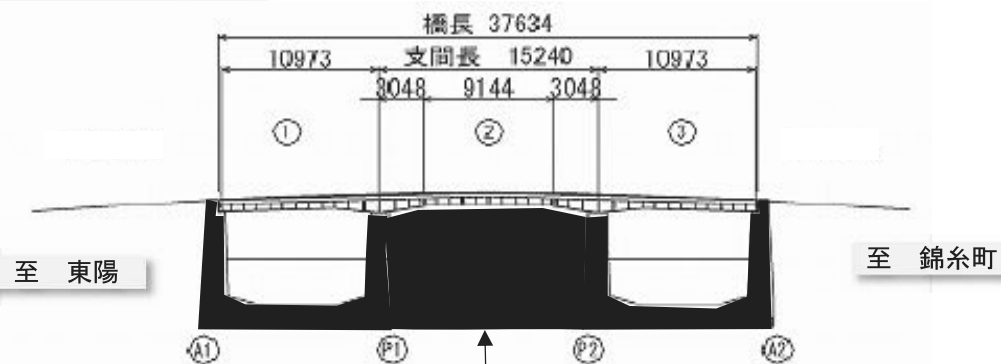
側 面 図
