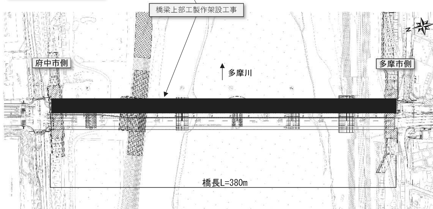
平 面 図
