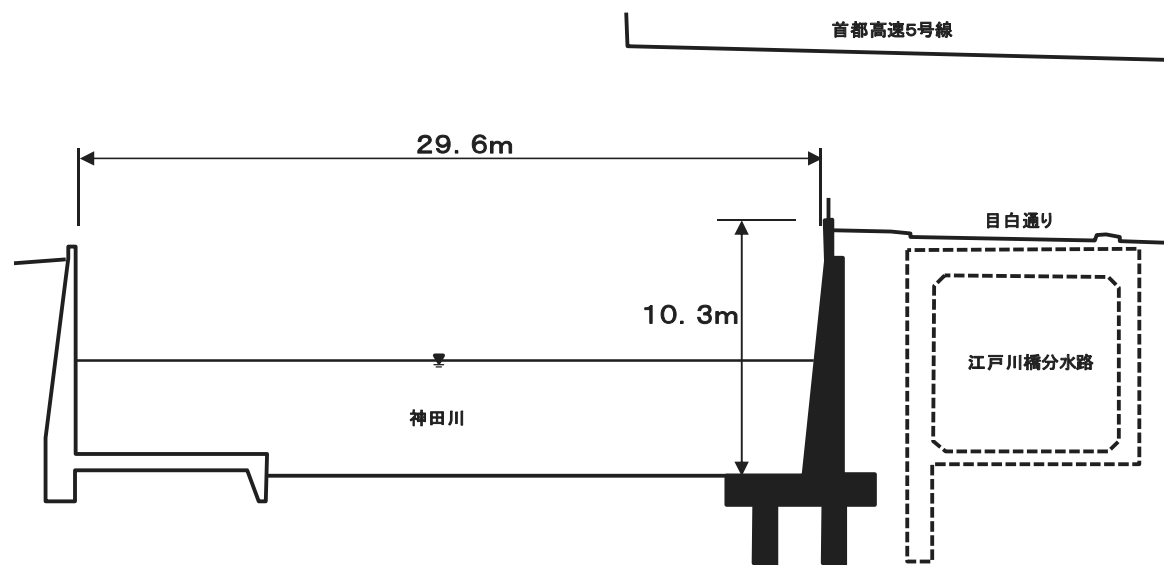
標準断面図
