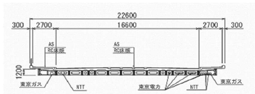
断 面 図
