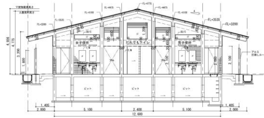
防災トイレ断面図（東西方向）
