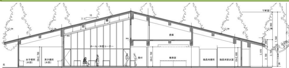
管理棟断面図（東西方向）
