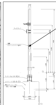
防犯カメラ参考図
