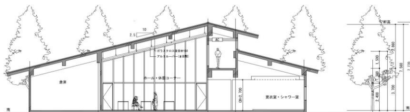
管理棟断面図（南北方向）
