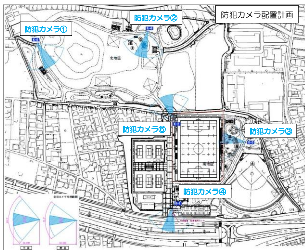
防犯カメラ参考図
