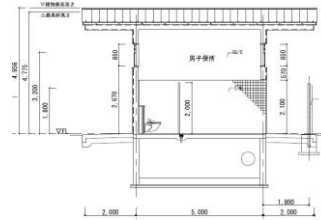
防災トイレ断面図（南北方向）
