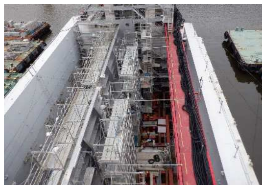
(施工状況：扉体組立)
