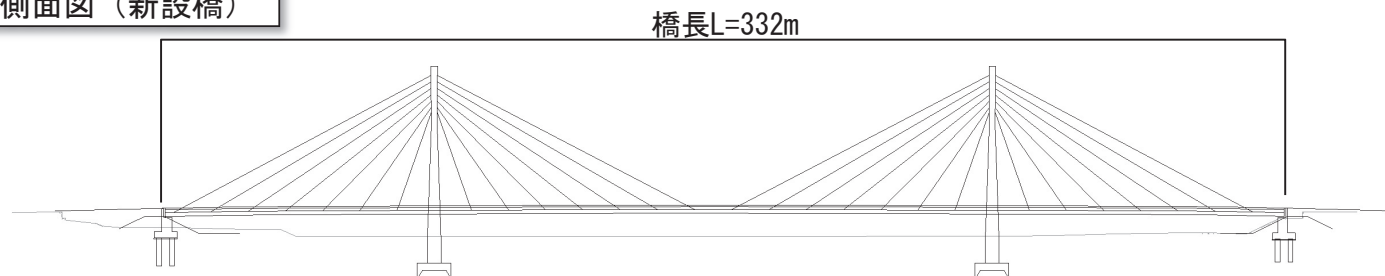
側面図（仮橋）
