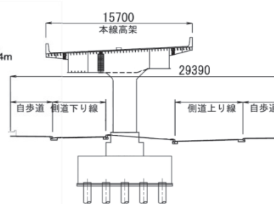
勝どき高架橋断面図
