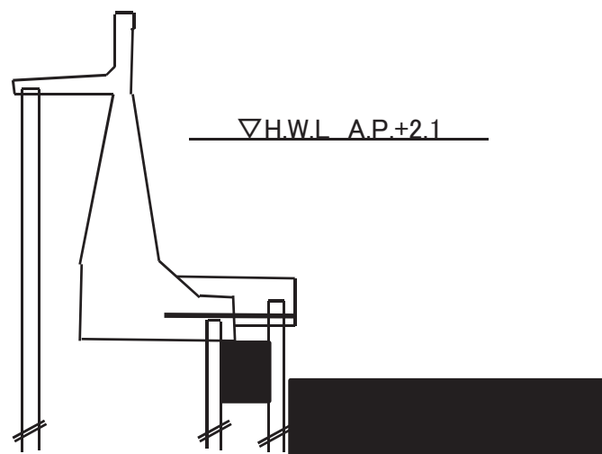
標準断面図
