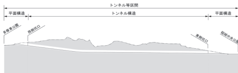
縦断面図
