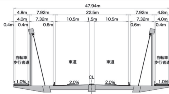
築地大橋断面図
