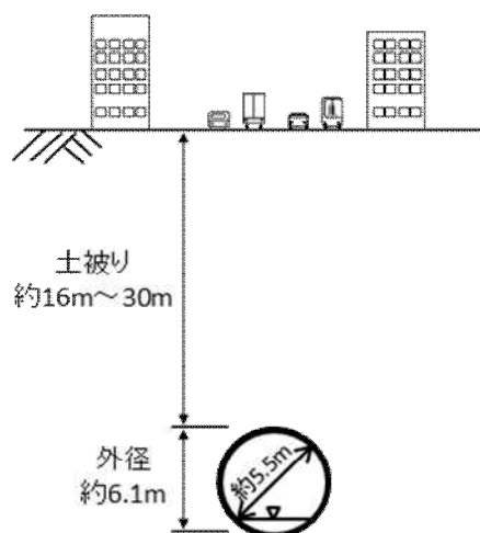
標準断面図
