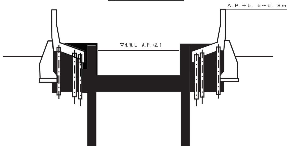
標 準 断 面 図
