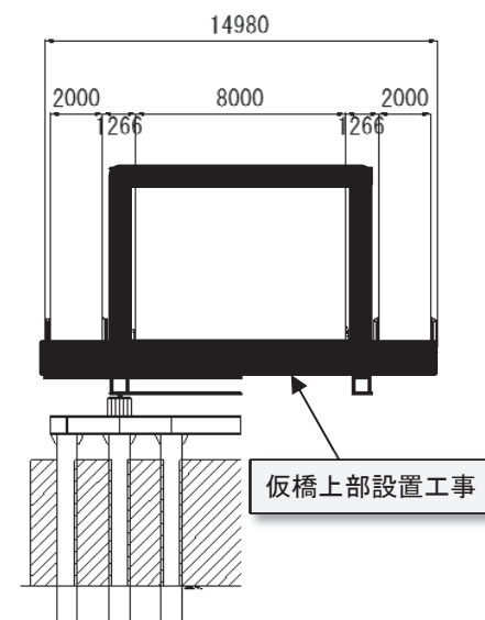
断面図（仮橋）
