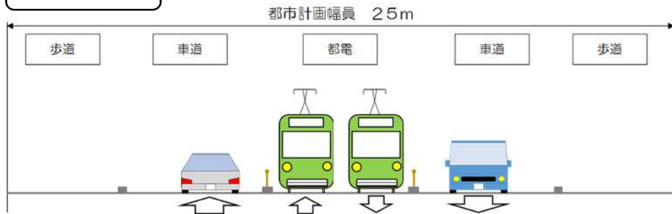
標準断面図
