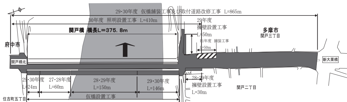
図-15 府中町田線（主18号 鎌倉街道）関戸橋
