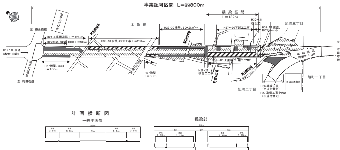
図-14 町田3・3・36号[旭町]（相原鶴間線）
