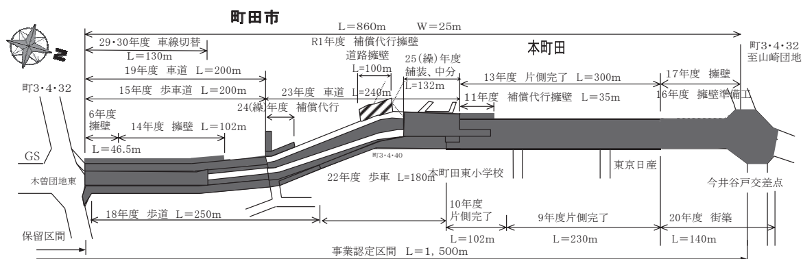
図－6 主要地方道府中町田線（主18号 鎌倉街道）本町田Ⅰ期
