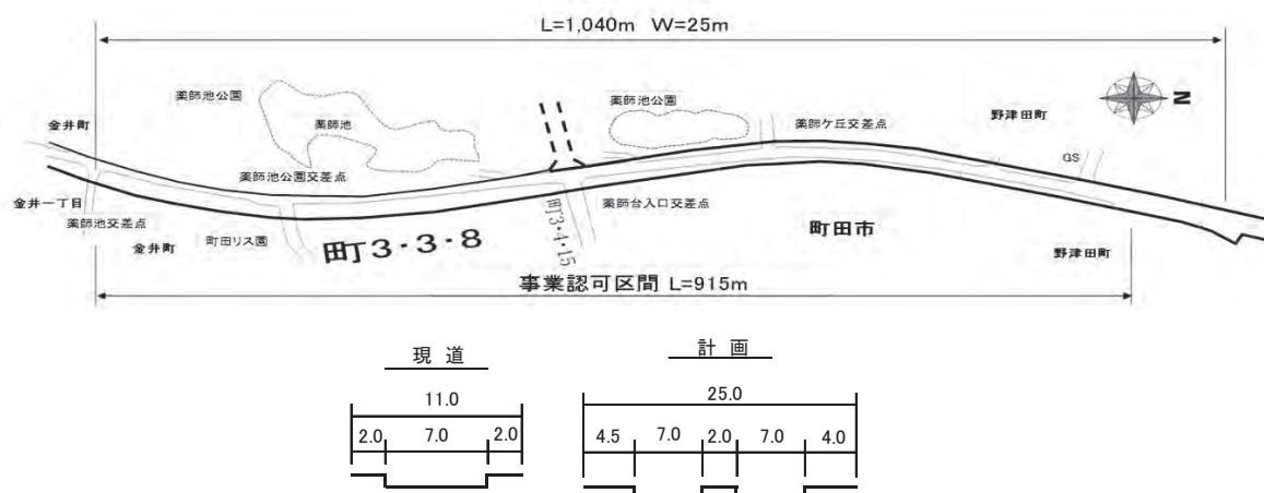
図－9 主要地方道府中町田線（主18号 鎌倉街道）薬師池Ⅱ期
