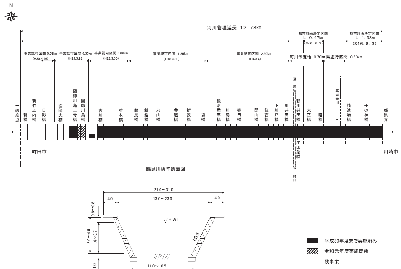
図-24 鶴見川
