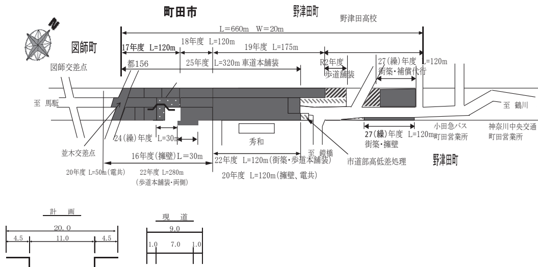
図－11 主要地方道相模原大蔵町線（主57号 芝溝街道）並木地区
