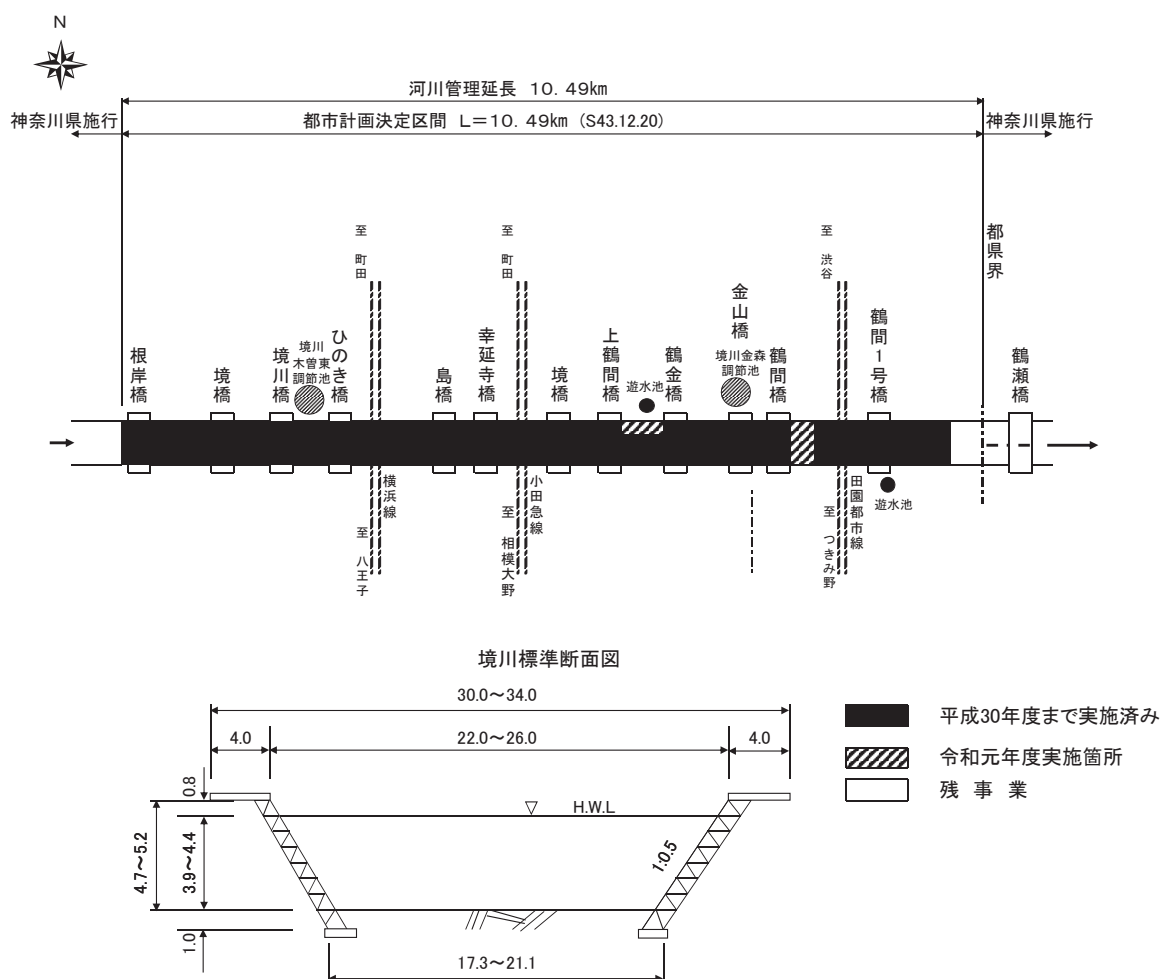
图-26 境川
