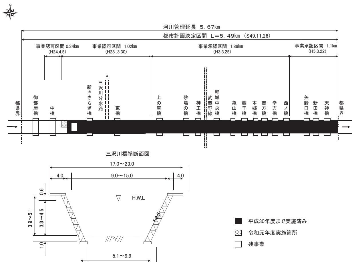
図-23 三沢川
