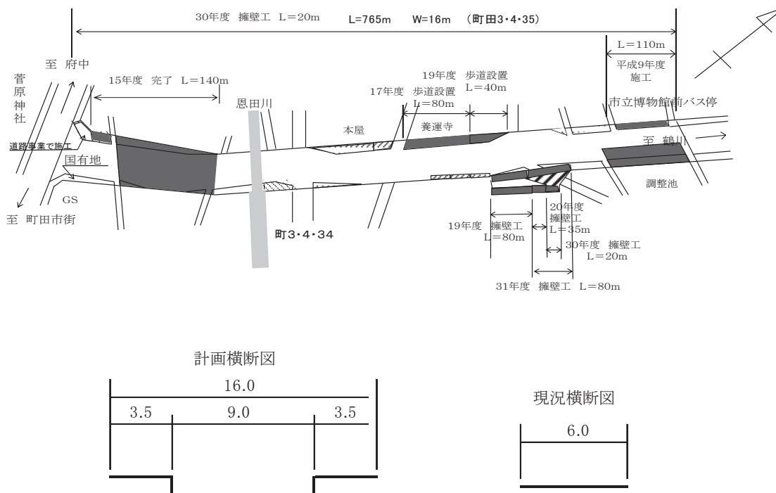
図-16 世田谷町田線（主3号 鶴川街道）玉川学園
