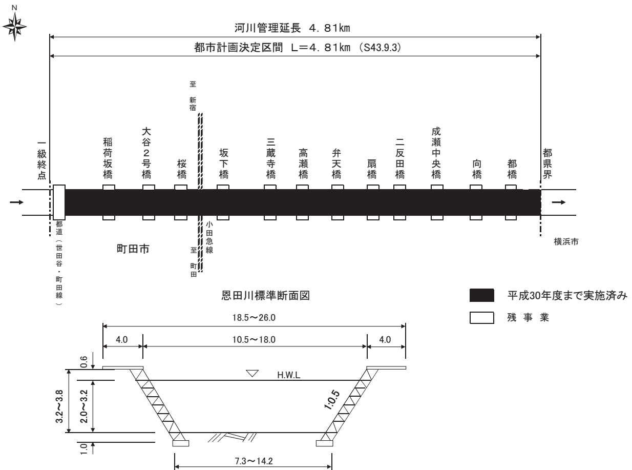
図-25 恩田川
