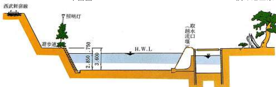
断面図
