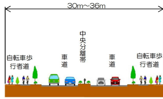
三鷹3・2・2標準断面
