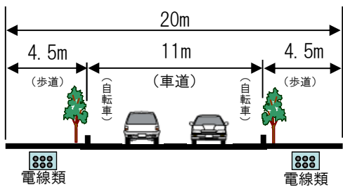
計画断面図
