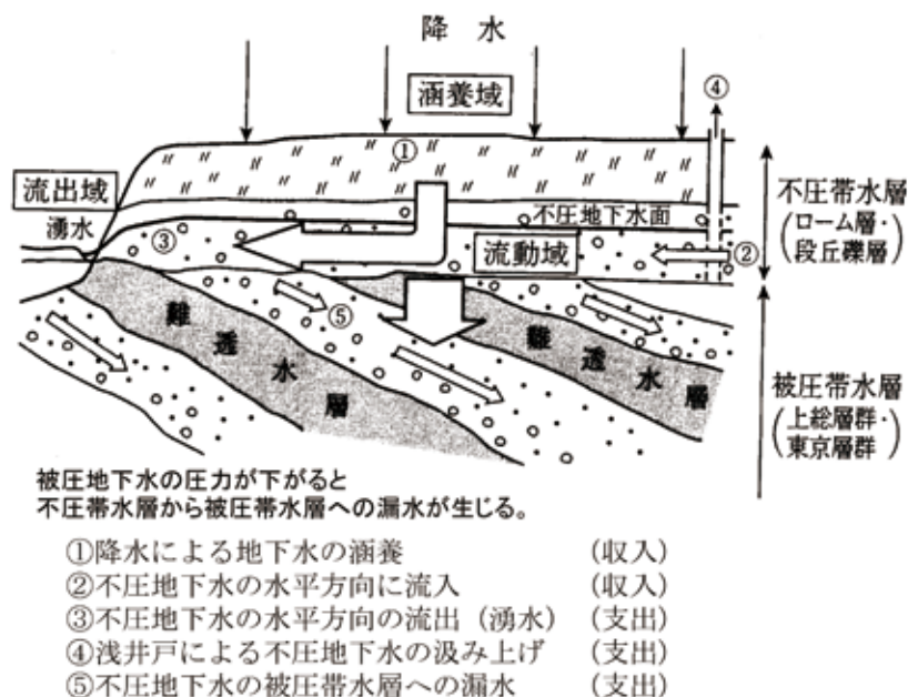
図—2. 洪積台地の湧水のしくみ
