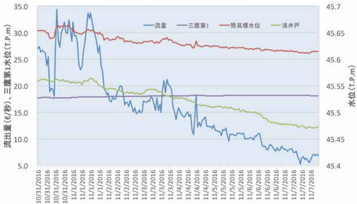
図ー5 ポンプ停止時の池流出量・水位
