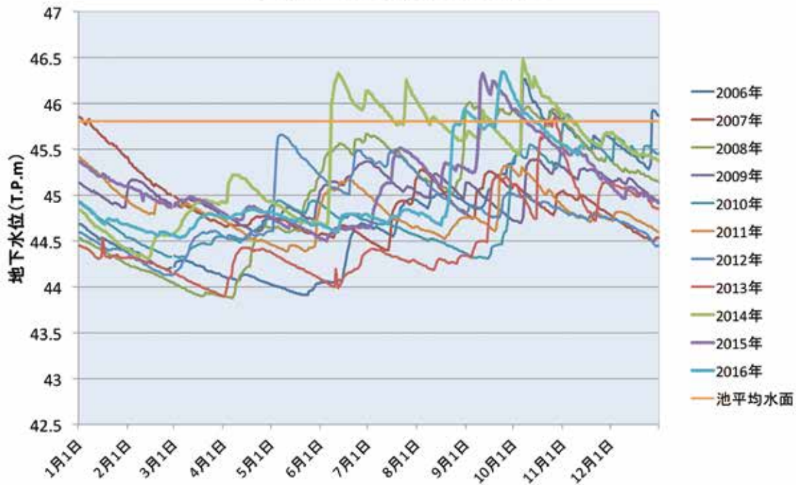
図-3. 井の頭浅井戸地下水位変動図（過去 11 年）
