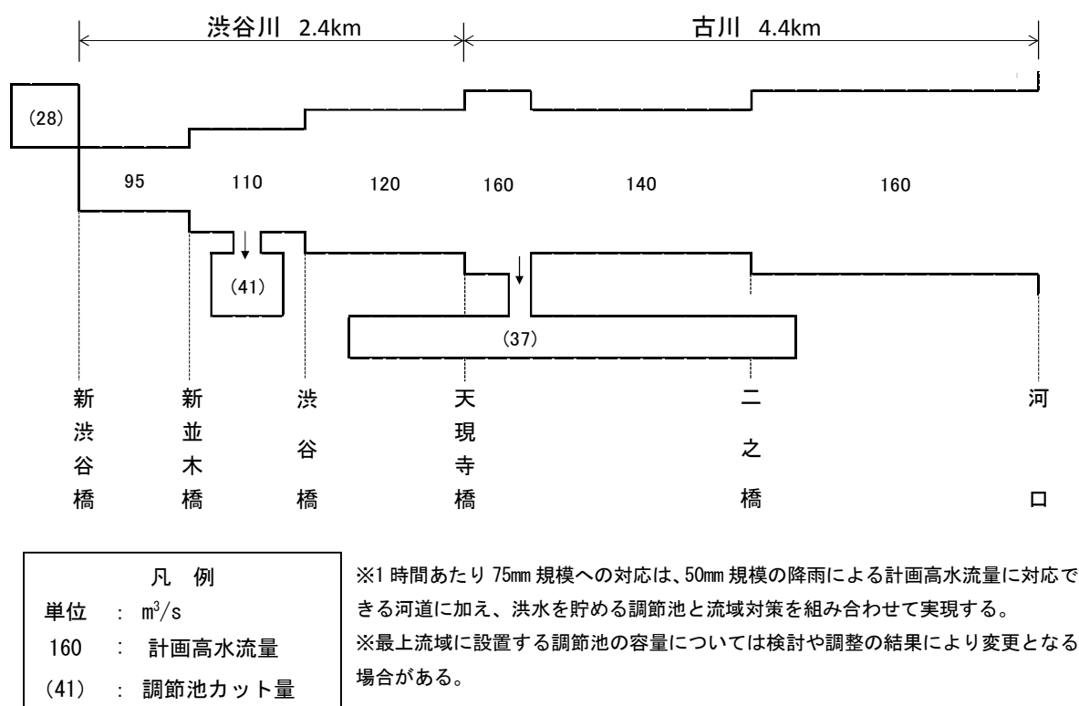
図3-1 渋谷川・古川流量配分図
