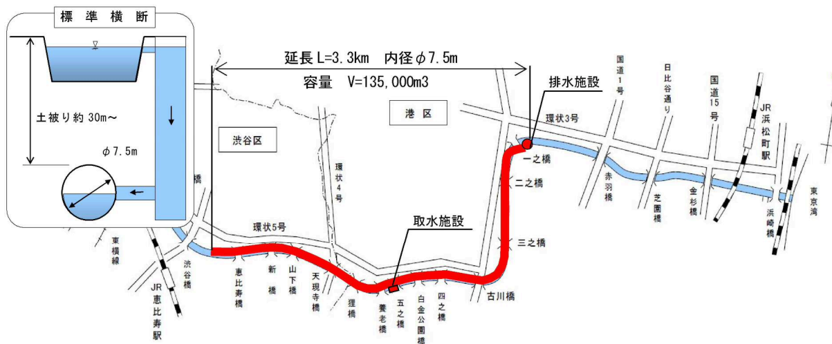
図 2-3 古川地下調節池概要
