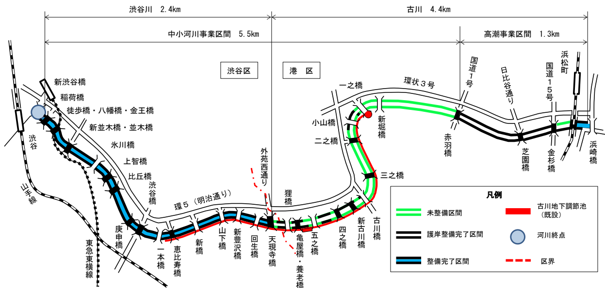
図2-2 渋谷川・古川河川整備概要図(平成29年度末)
