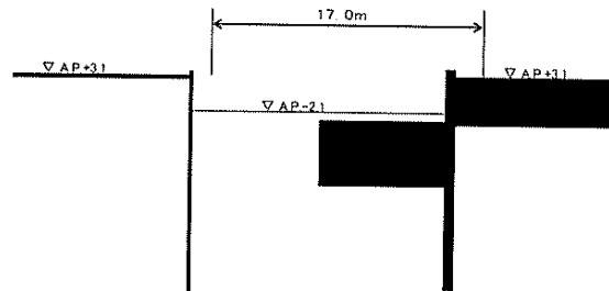
標準断面図
