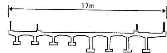
断 面 図
