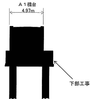
橋台断面図
