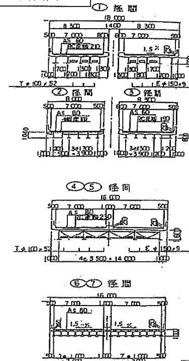
断面図
