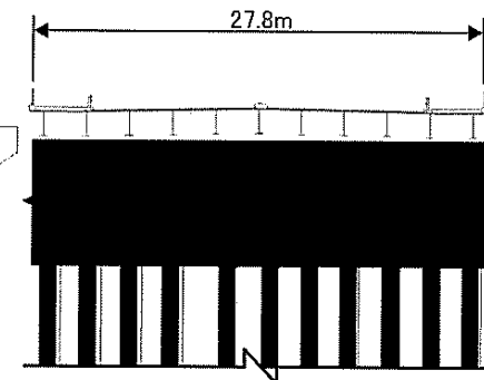
新橋断面図
