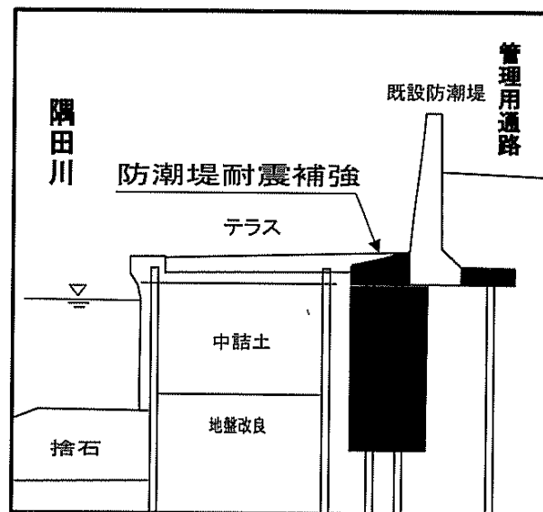
標準断面図
