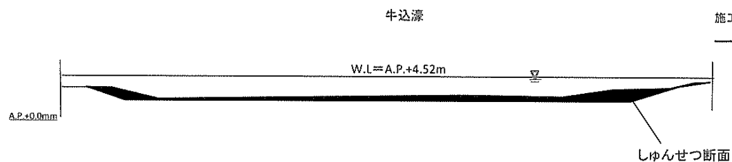
標準断面図
