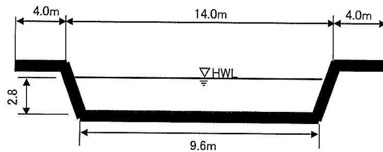
標 準 断 面 図
