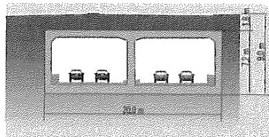
トンネル断面図
