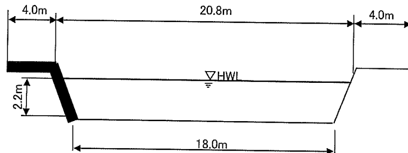
標 準 断 面 図
