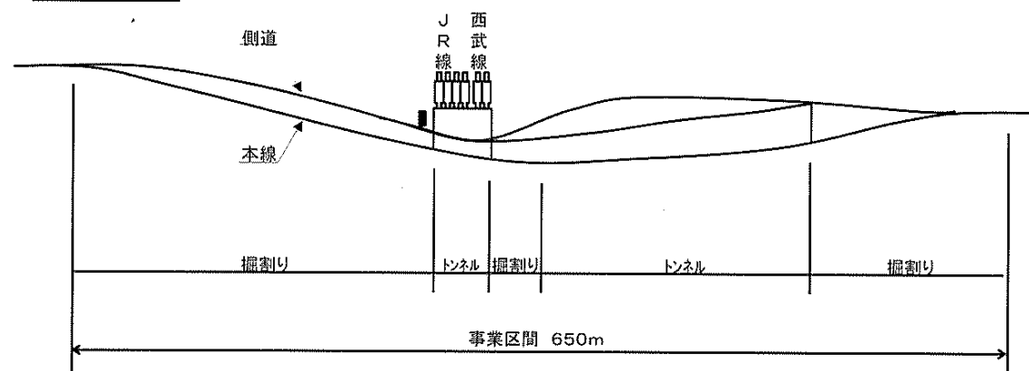
側面図
