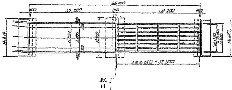
平面図
