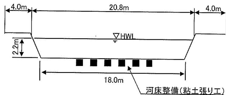
標 準 断 面 図
