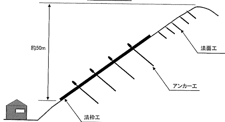
標準断面図
