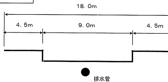
断面図
