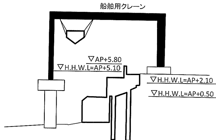
標 準 断 面 図
