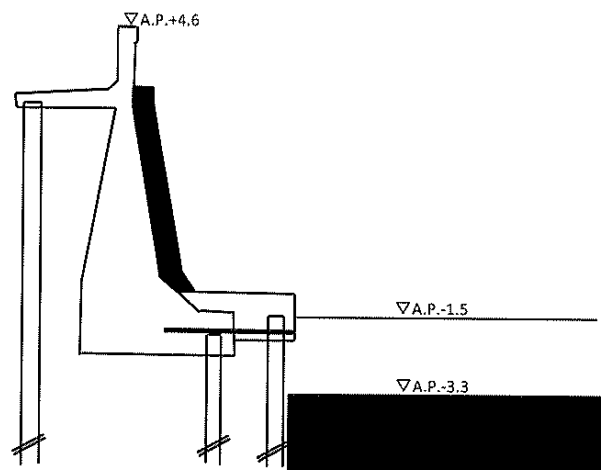
標準断面図
