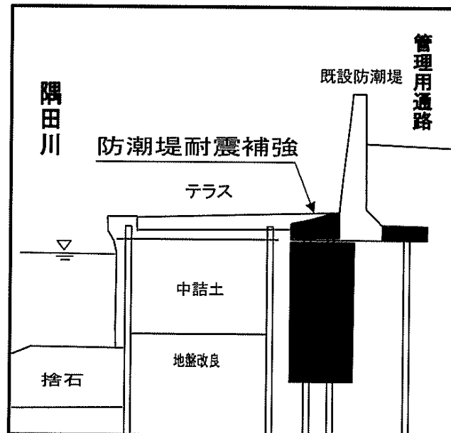
標準断面図
