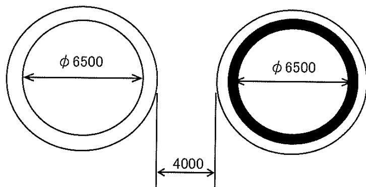
標準断面図
