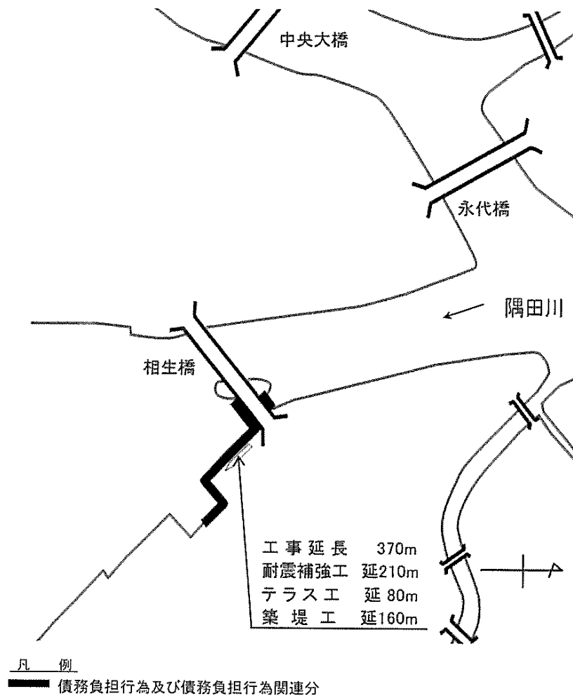
平面図
