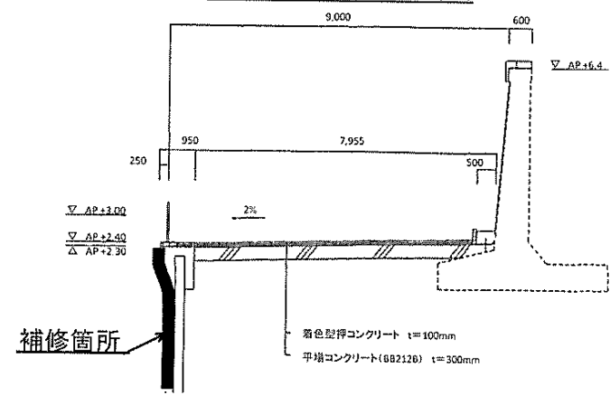
標 準 断 面 図
