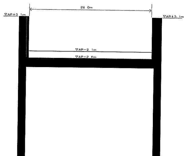
標準断面図
