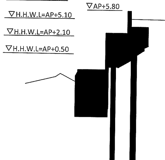
標 準 断 面 図
