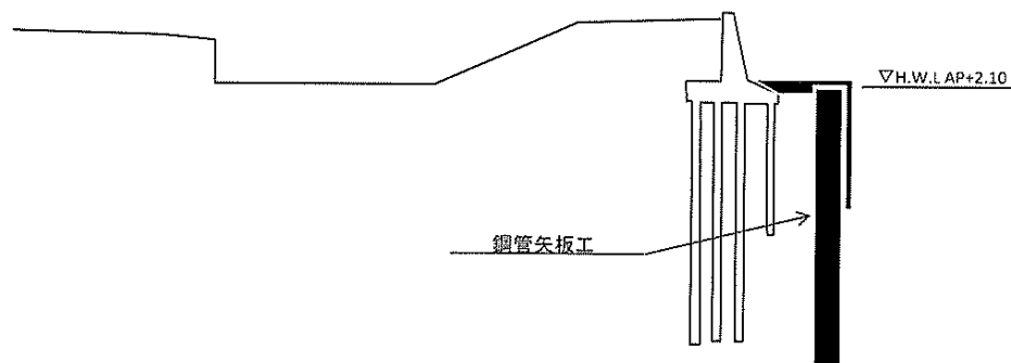
標準断面図
