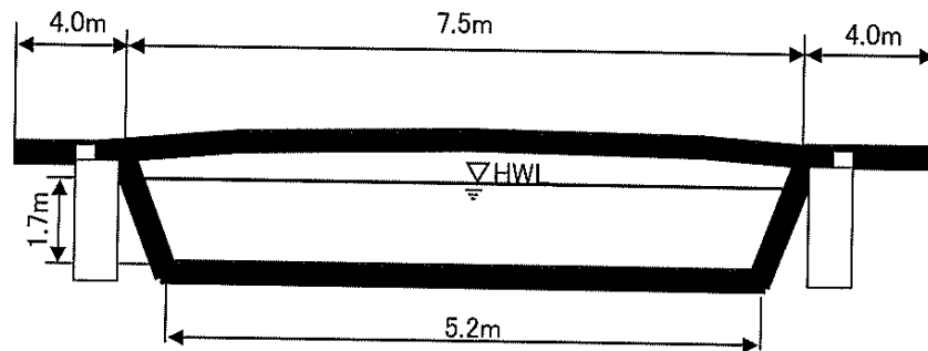
標 準 断 面 図
