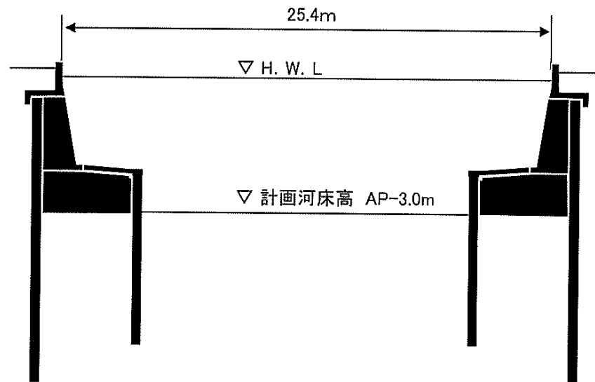
標 準 断 面 図
