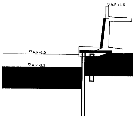
標準断面図
