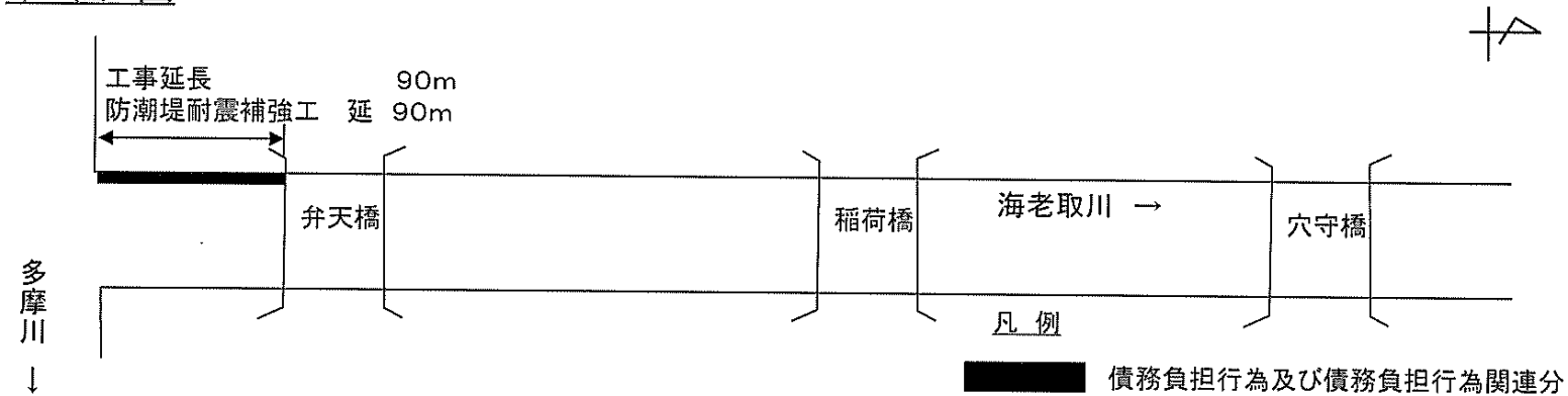
平面図
