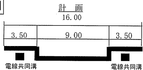
断面図
