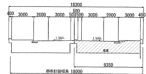
断面図(幅員構成未定)
