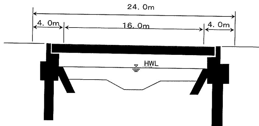
標 準 断 面 図
