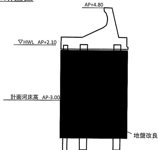
標準断面図
