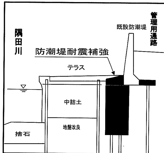
標準断面図
