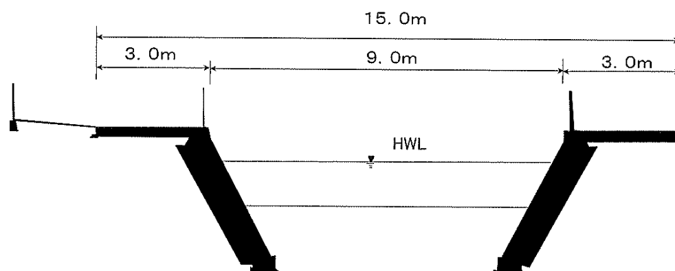
標 準 断 面 図
