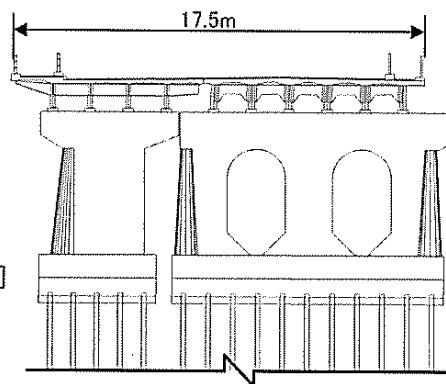
旧橋断面図
