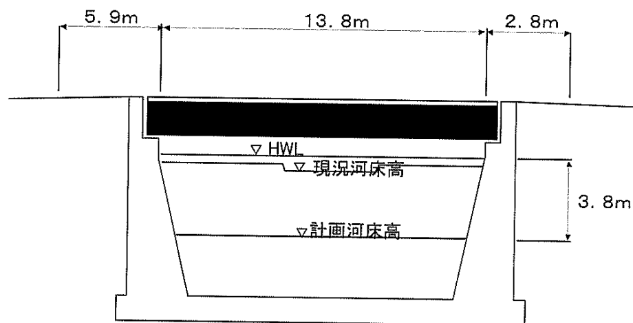
標 準 断 面 図
