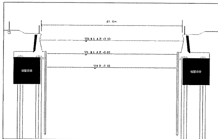
標準断面図
