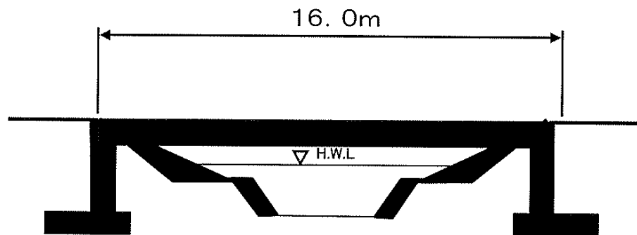
標準断面図
