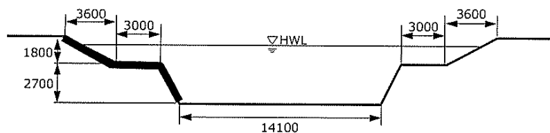
標準断面図
