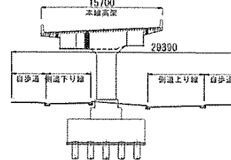
勝どき陸橋断面図
