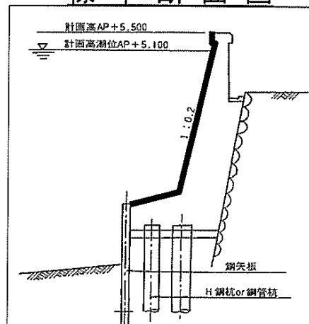
標 準 断 面 図
