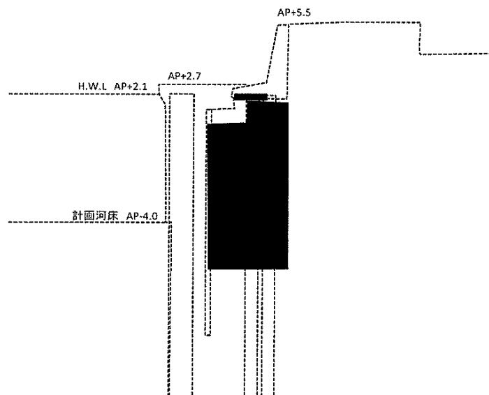
標準断面図
