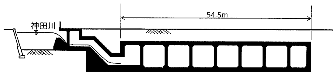
標 準 断 面 図
