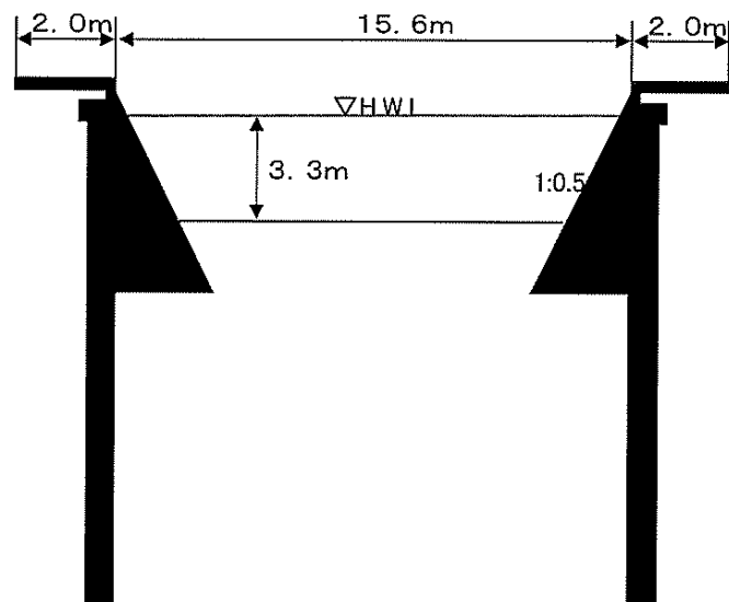
標準断面図
