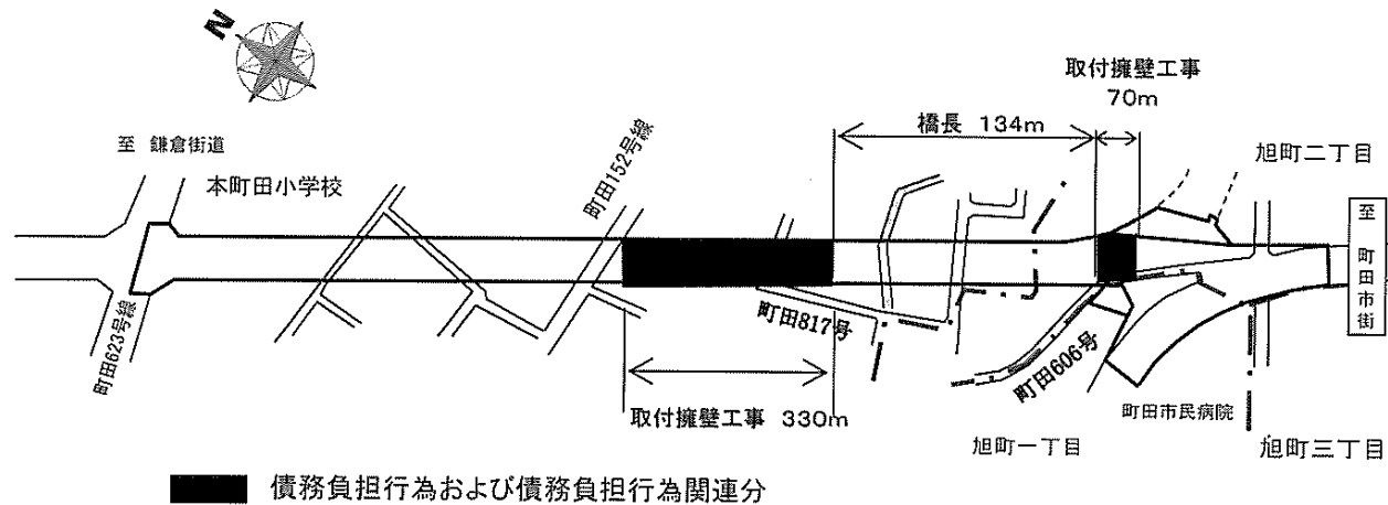
平面図
