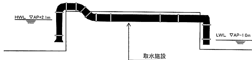
標準断面図
