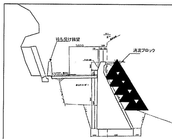
標準断面図
