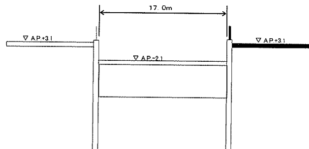
標準断面図
