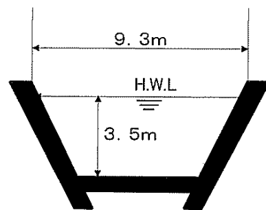
標準断面図
