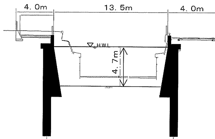
標 準 断 面 図
