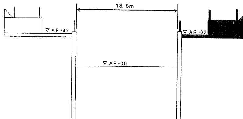
標準断面図
