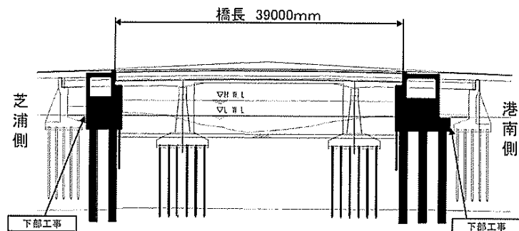
側 面 図
