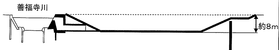
標 準 断 面 図
