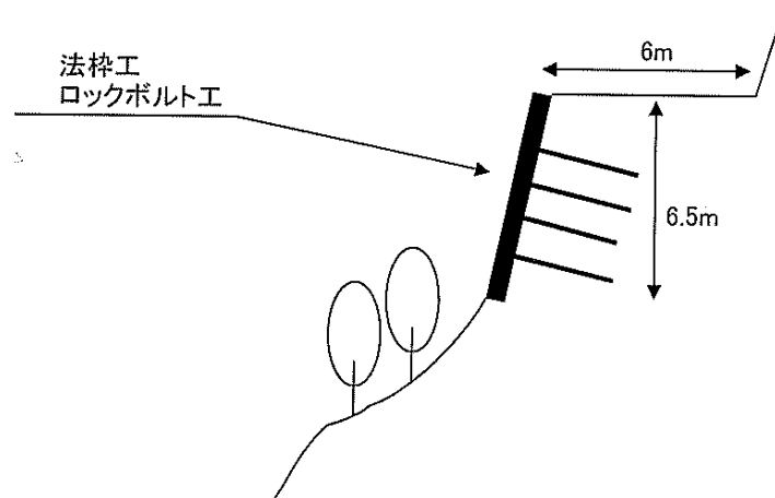
断面図
