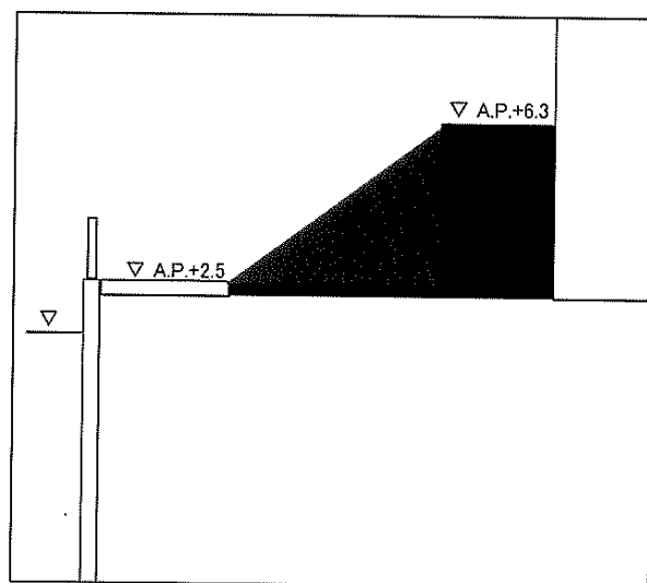
標準断面図
