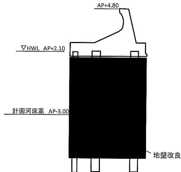
標準断面図
