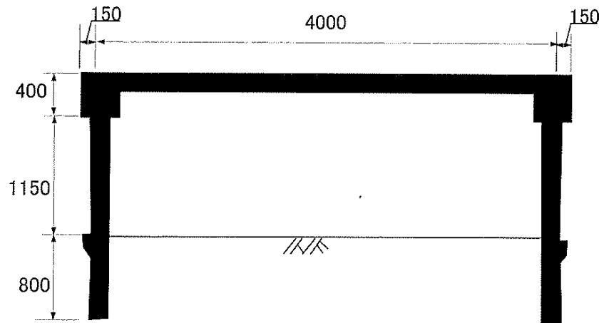
標準断面図
