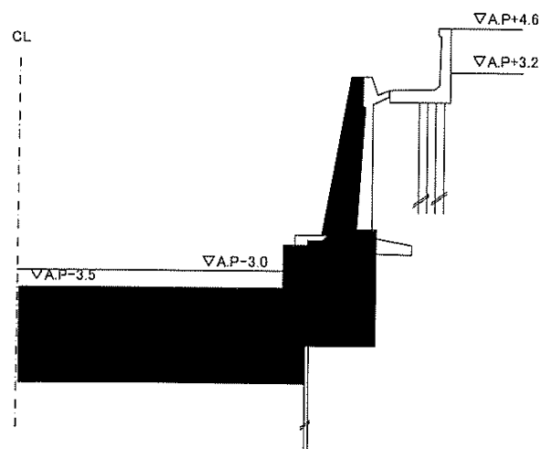
標準断面図
