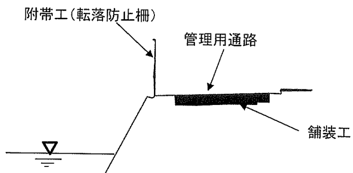
標 準 断 面 図
