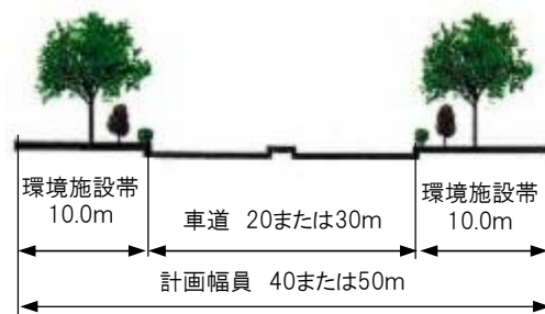
標準断面図
