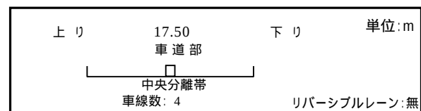
横断構成図
