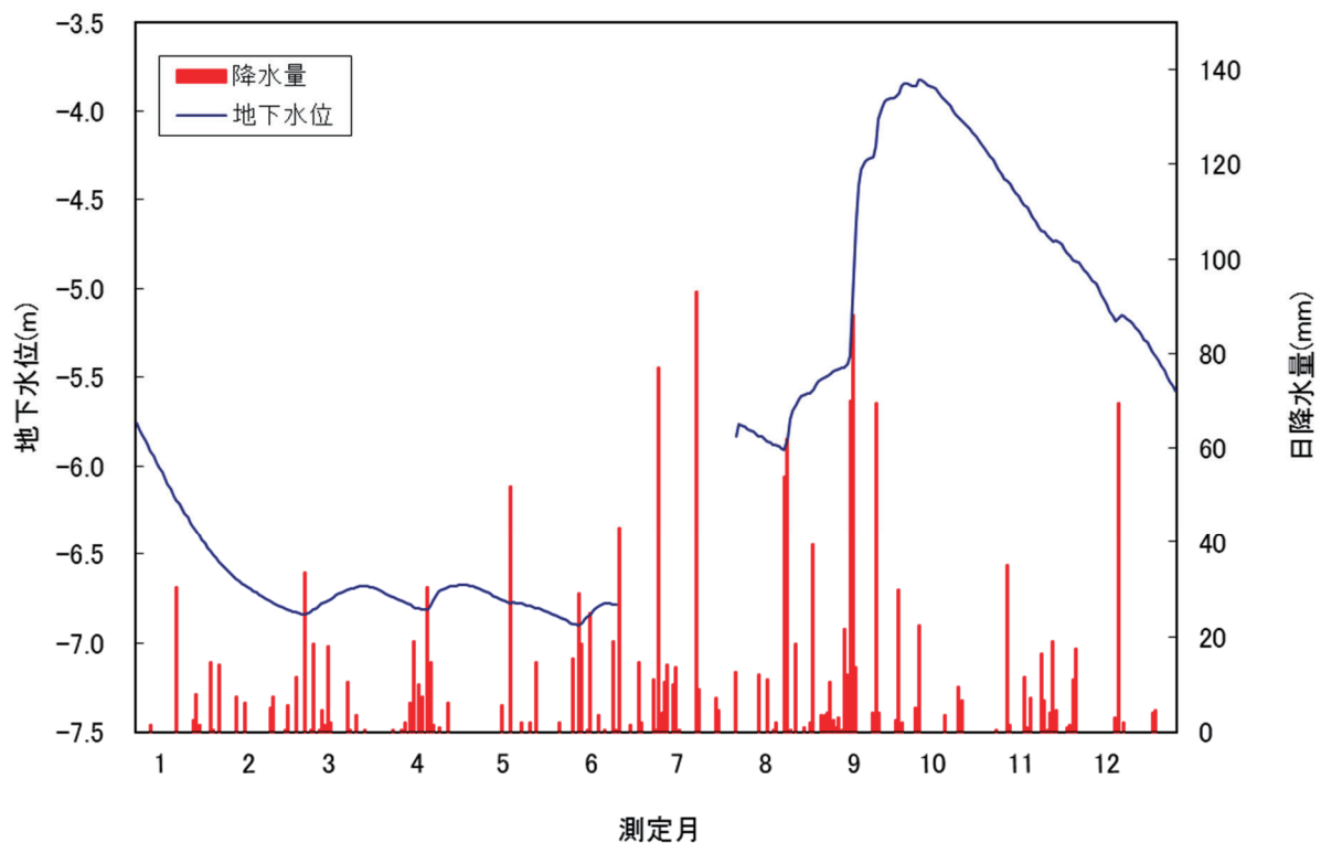
図一 8 平成 27 年地下水位と降水量 ⑥小金井市 貫井南町
