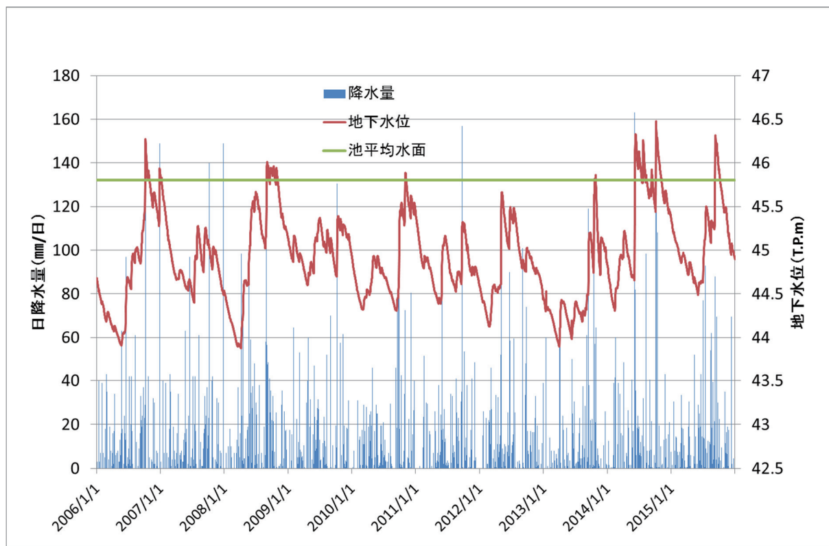
図－9 井の頭公園経年地下水位変動図（過去10年）
