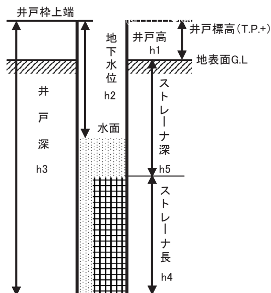
図－２ 地下水位測定要素
