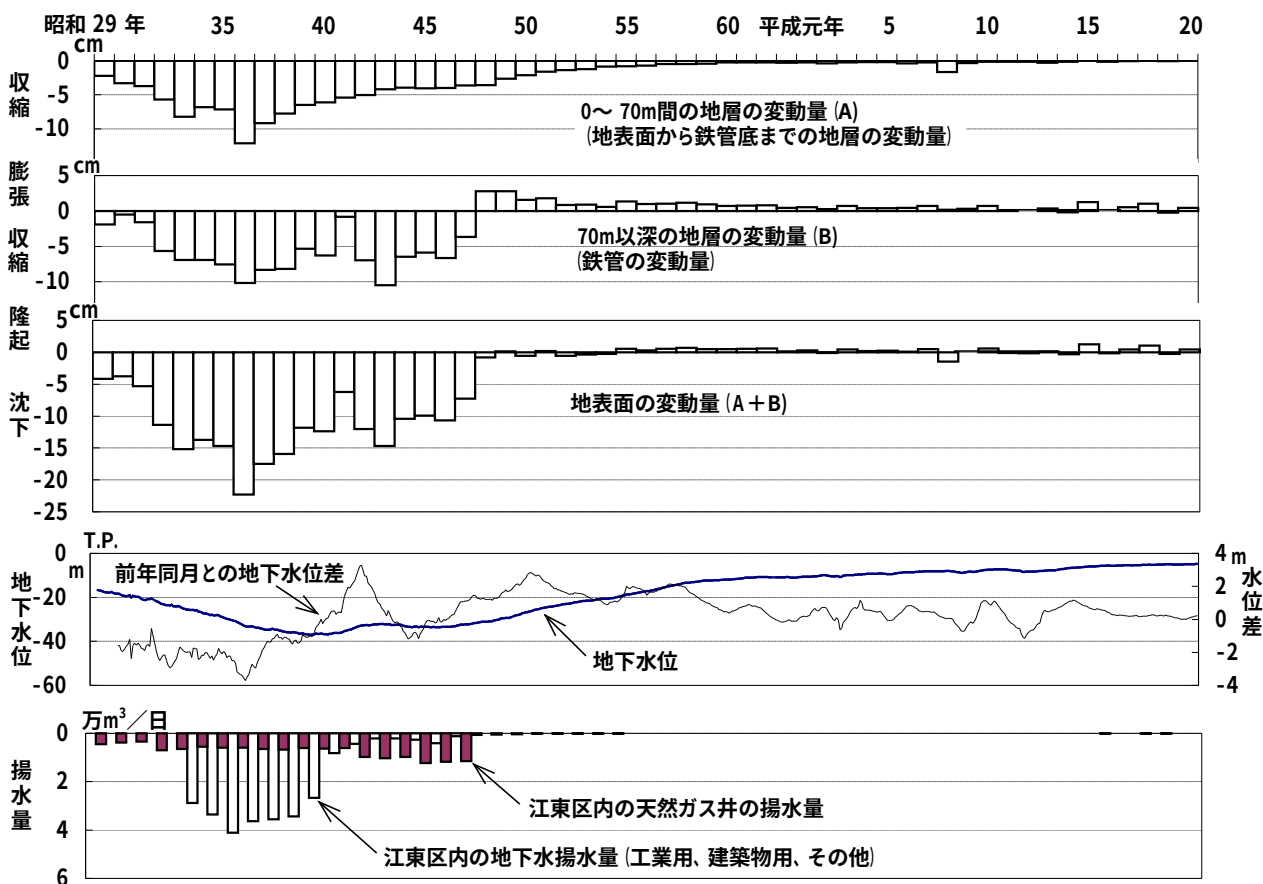
図-17 南砂町第1観測井(70m井)における地盤変動量と地下水位との関係
