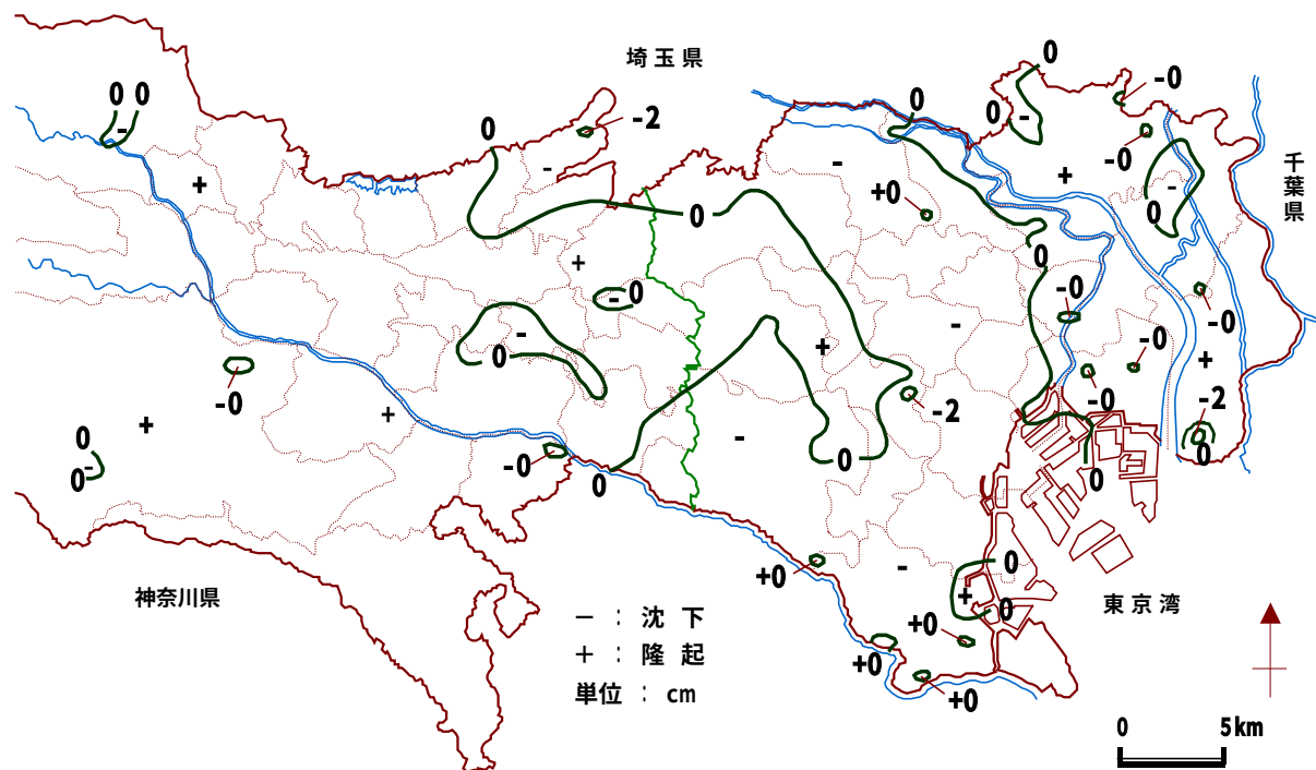
図-3 最近5年間の地盤変動量図（平成16年～平成20年）
