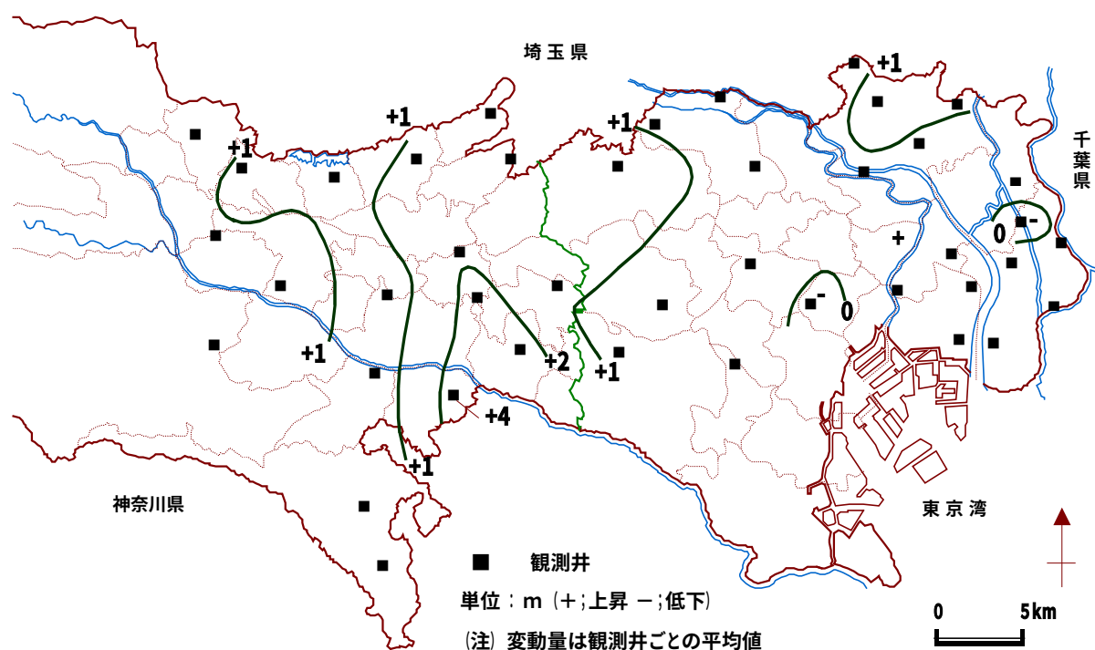
図-6 平成20年の地下水位変動量図
