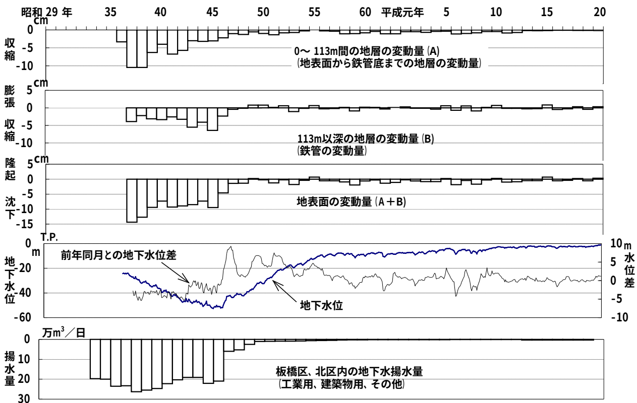
図-18 戸田橋第2観測井(113m井)における地盤変動量と地下水位との関係
