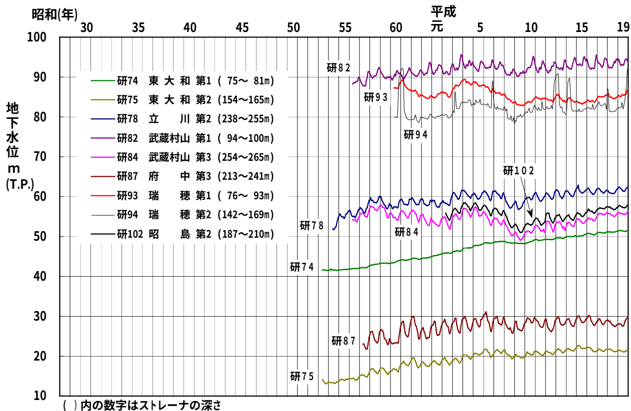
図-12 主な観測井の地下水位変動図（東大和市、武蔵村山市、瑞穂町、昭島市、立川市、府中市）
