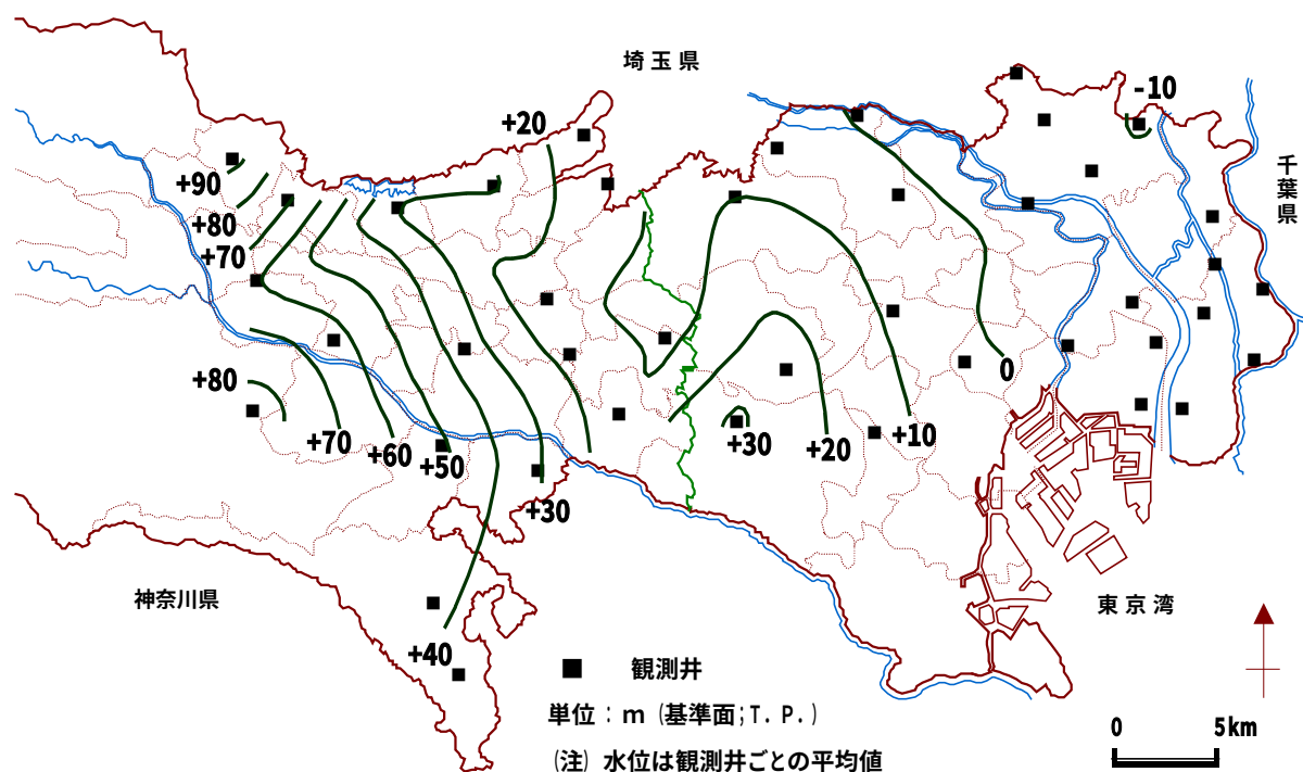
図-5 平成20年末の地下水位等高線図
