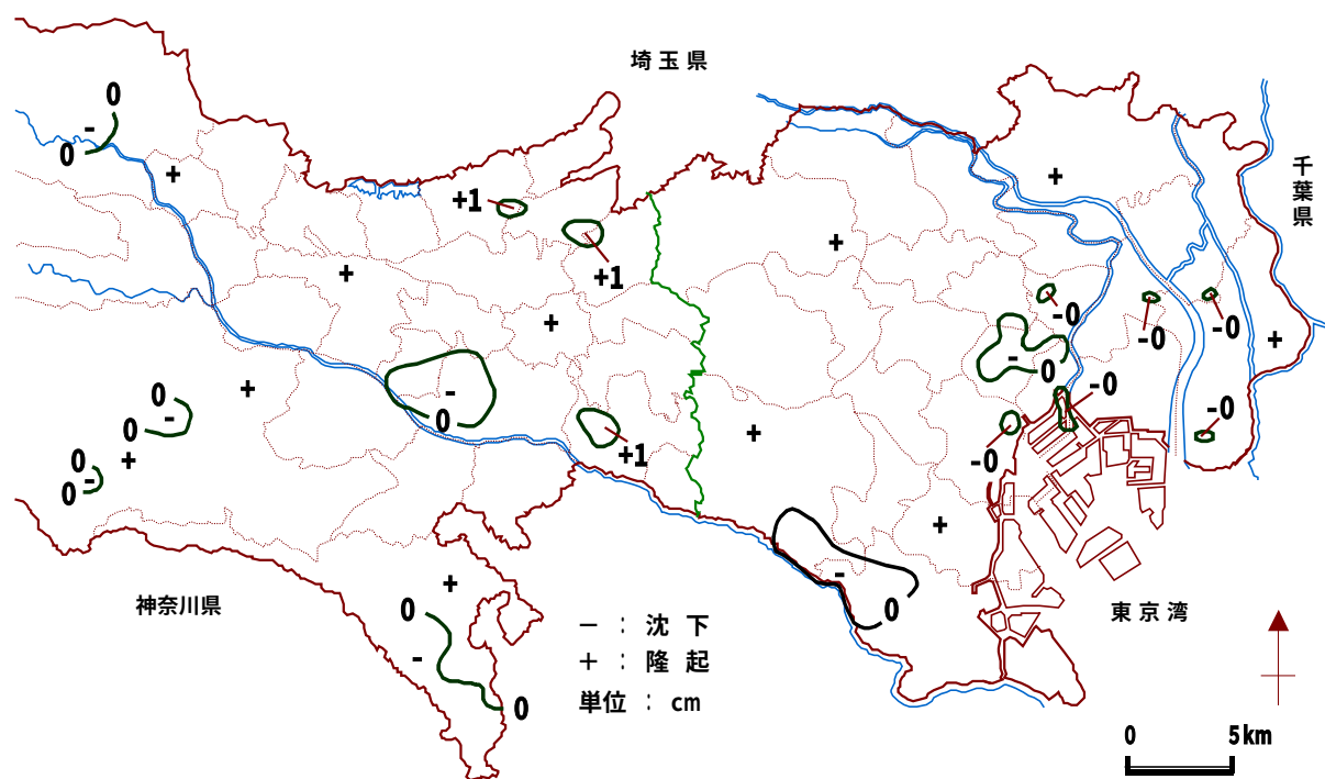
図-2 平成20年の地盤変動量図
