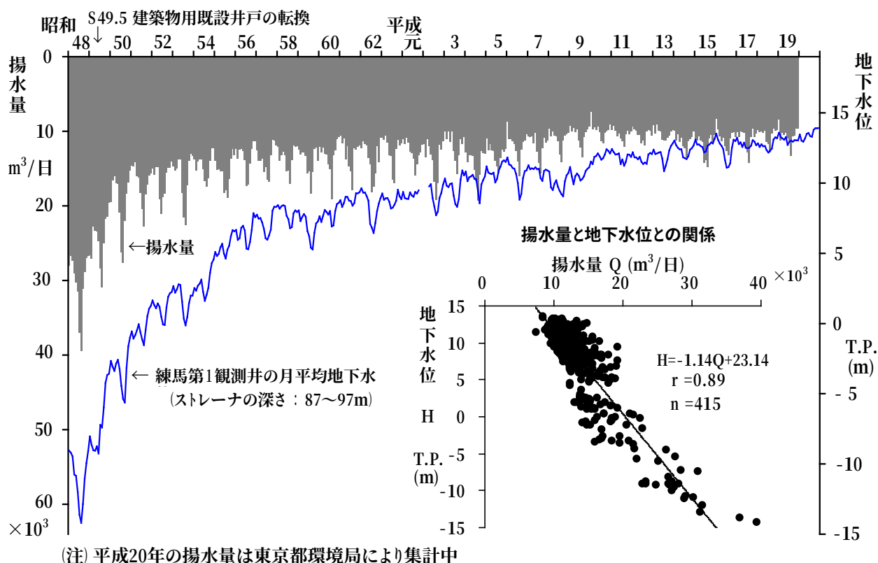
図-14 練馬区内の揚水量と地下水位との関係
