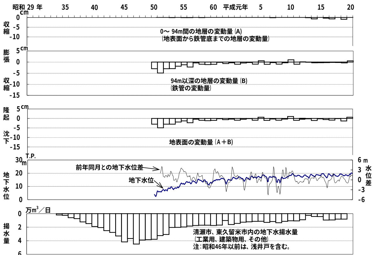
図-20 清瀬第1観測井(94m井)における地盤変動量と地下水位との関係
