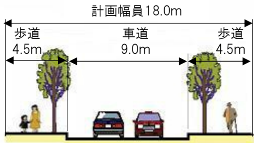
標準断面図
