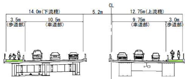
標準断面図
