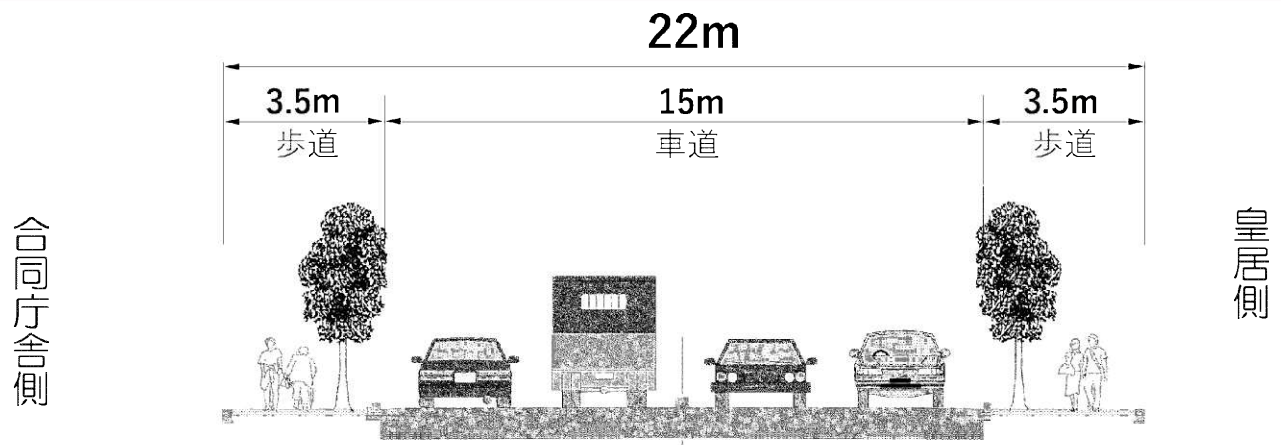
標準現況断面図
