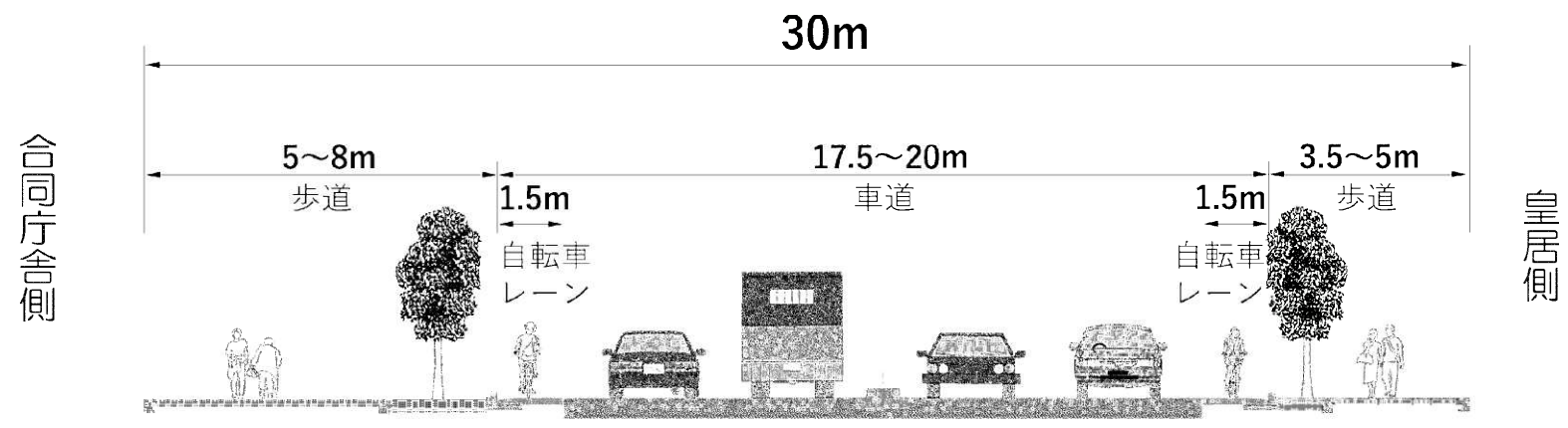
計画断面図
