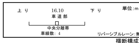
横断構成図
