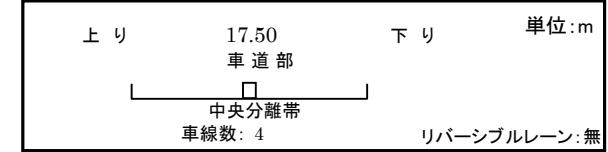
横断構成図
