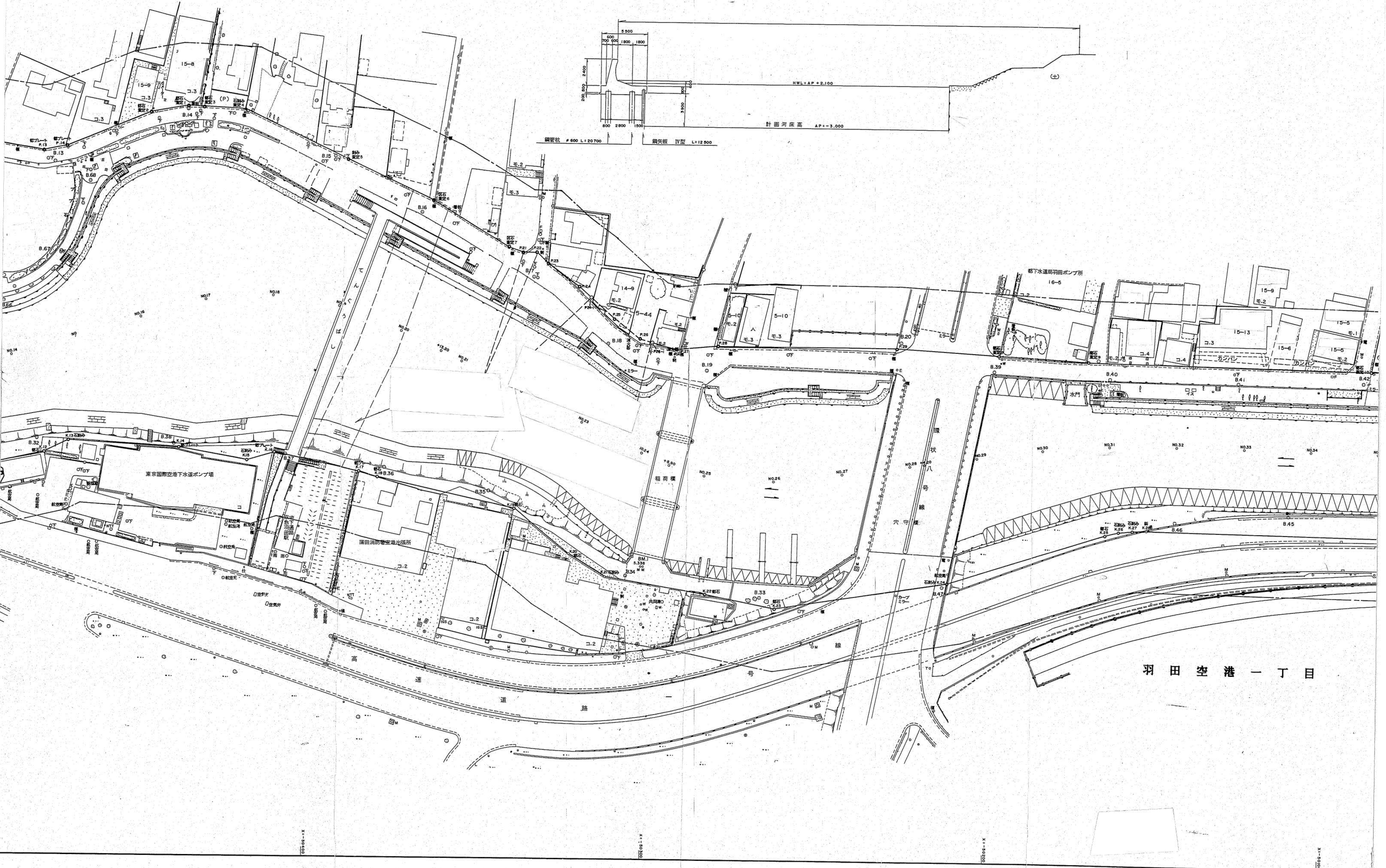
標準断面図 S = 1 : 200 (NO.22)
